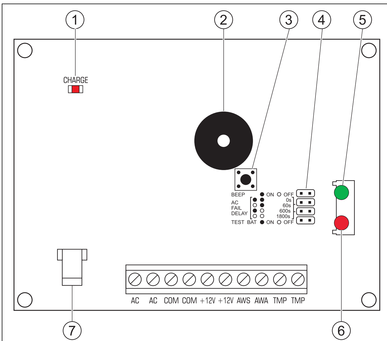
Rys. 1. Widok płytki elektronicznej.
