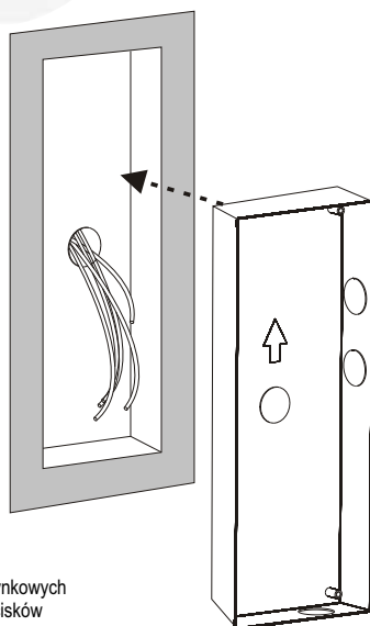
puszka podtynkowa
