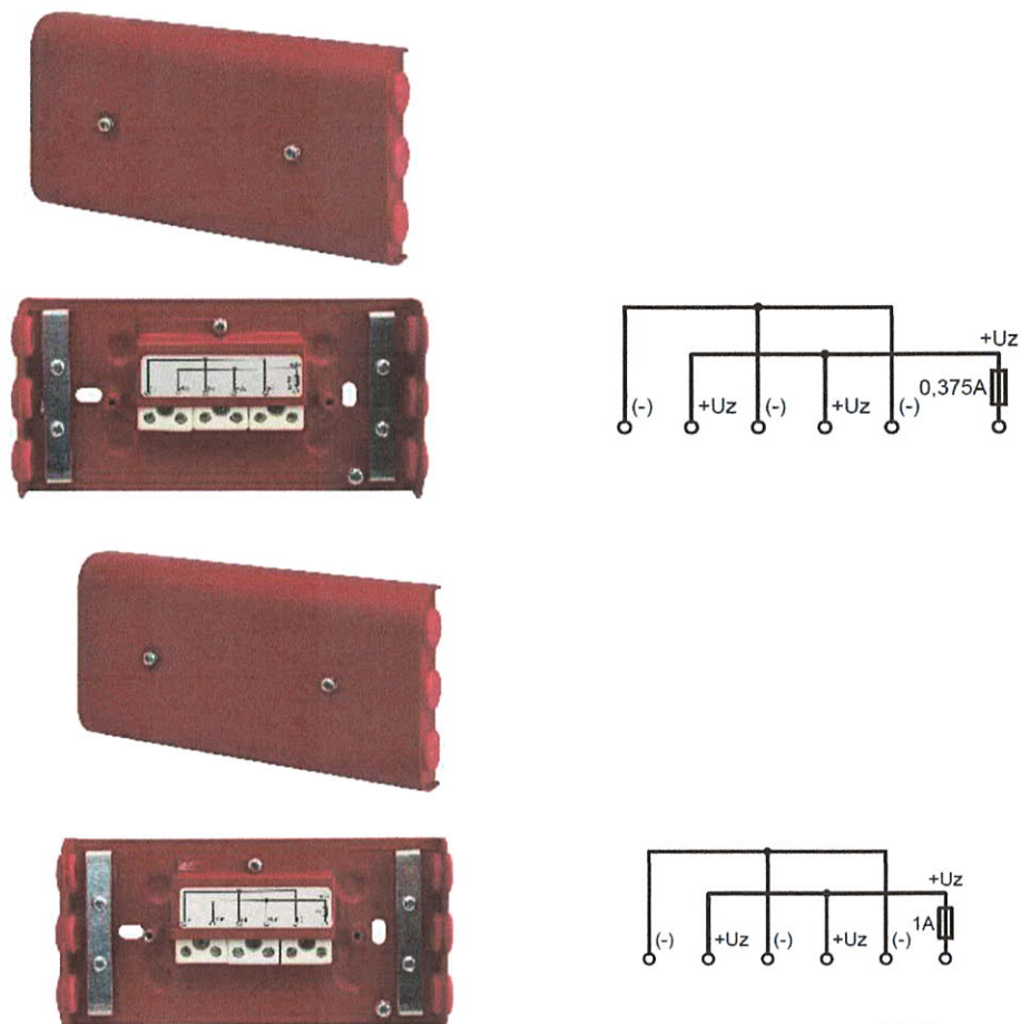
Rysunek 1 Puszki typu AWOZ-125P oraz AWOZ-125P1A
