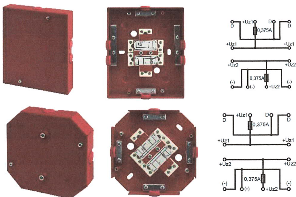
Rysunek 3 Puszki typu AWOZ-225P oraz AWOZ-225S
