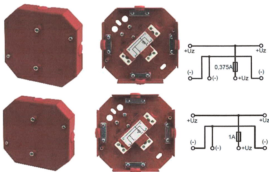
Rysunek 2 Puszki typu AWOZ-125S oraz AWOZ-125S1A
