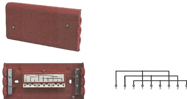
Puszka typu AWOP-360PR
