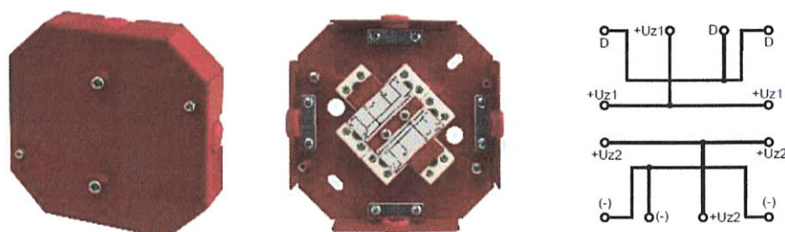
Puszka typu AWOP-425SR
