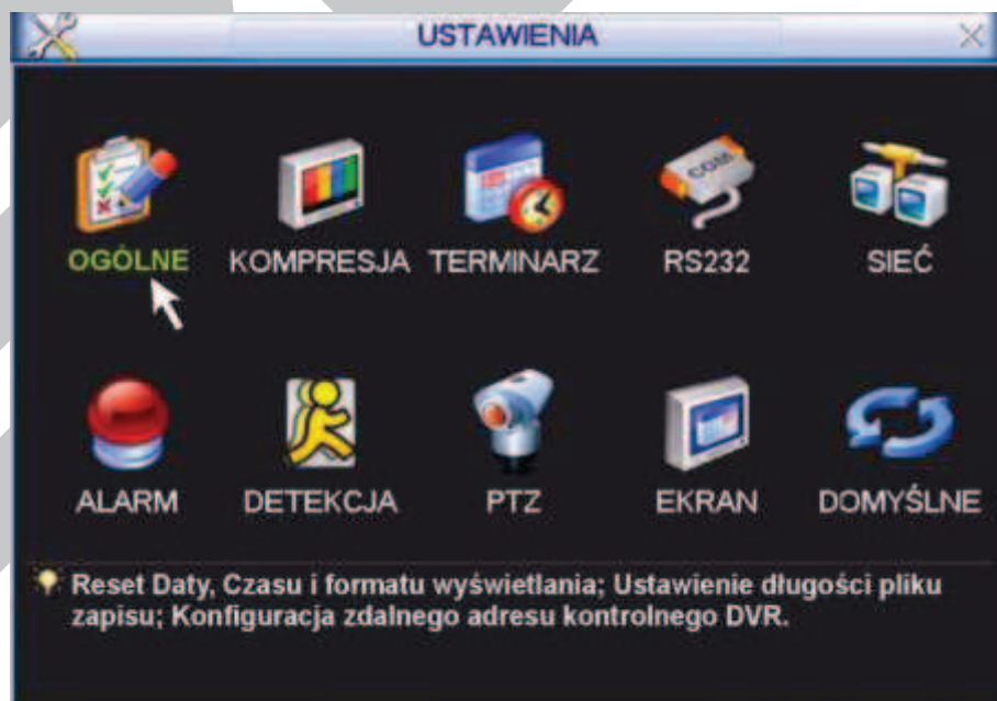
Rys. 5-2. Menu Ustawienia.
