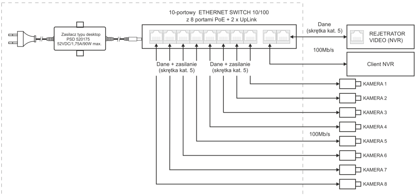
Rys. 1. Schemat blokowy.
