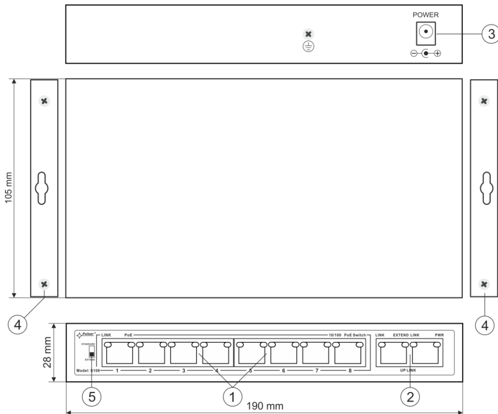
Rys. 2. Widok switch'a.
