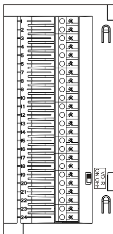
Terminal przyłączeniowy monitora
