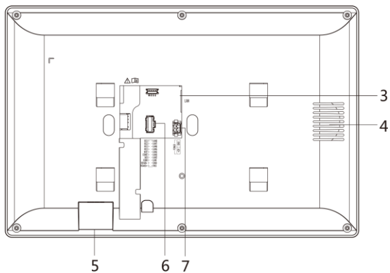
Rysunek 2-2 Tyłny panel
