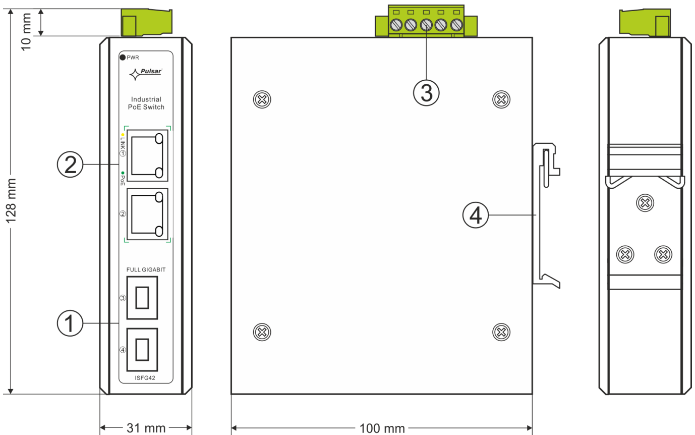
Rys. 2. Widok switch'a.
