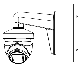
DS-1276ZJ-SUS Mocowanie narożne
