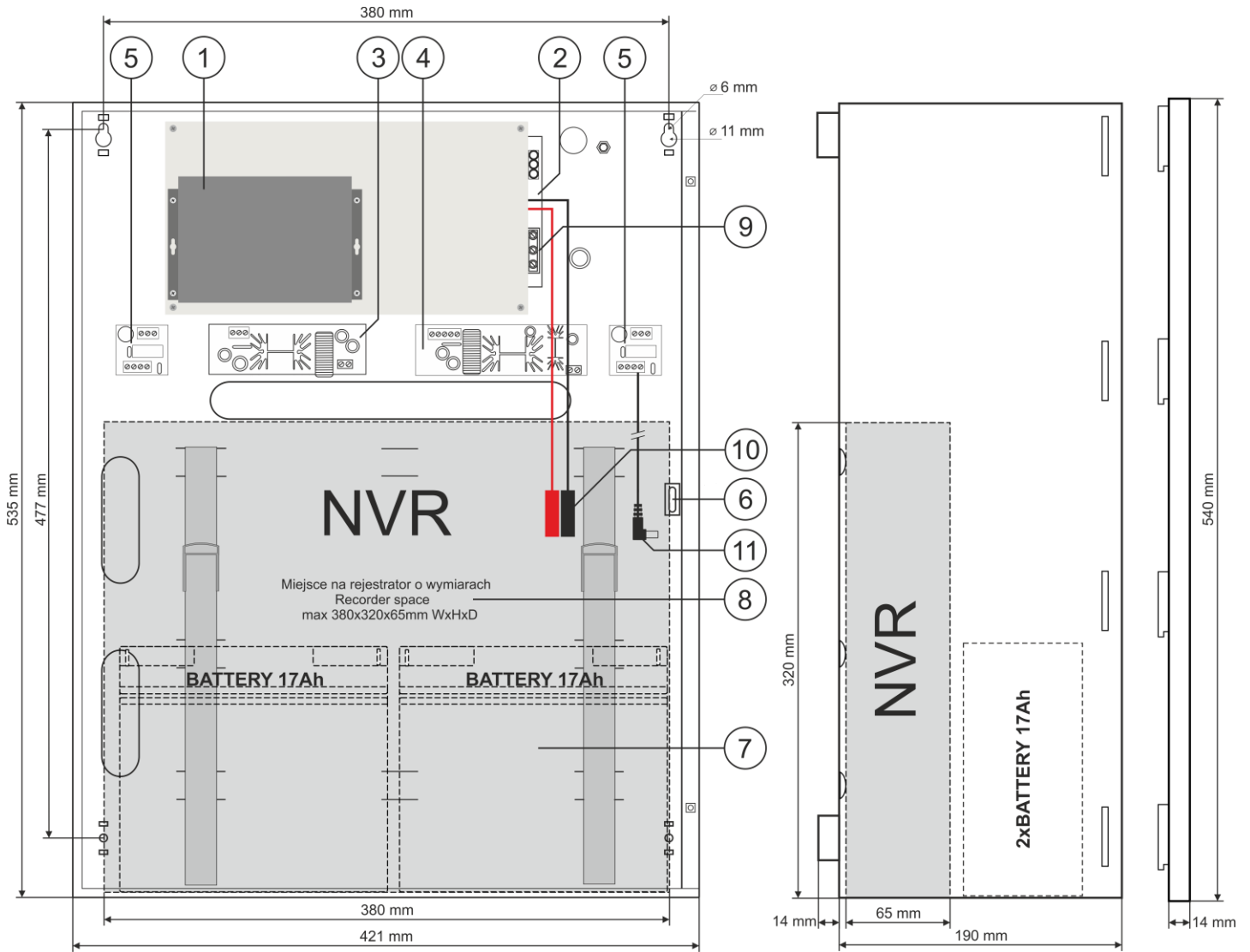
Rys. 2. Widok obudowy.
