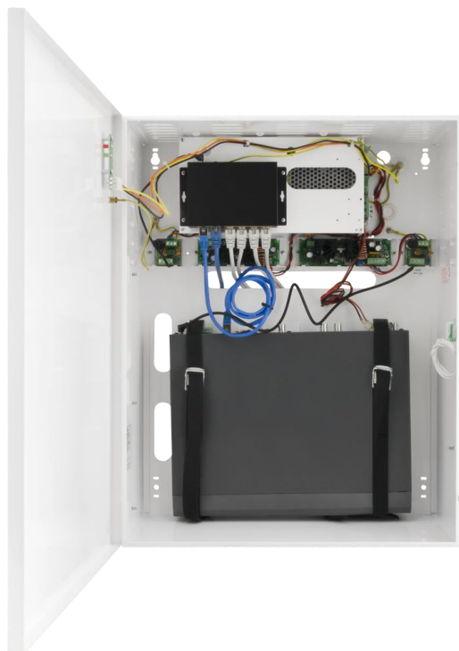
Przykładowy montaż S64-CRB z akumulatorami i rejestratorem. (zestaw nie zawiera rejestratora i akumulatorów)
