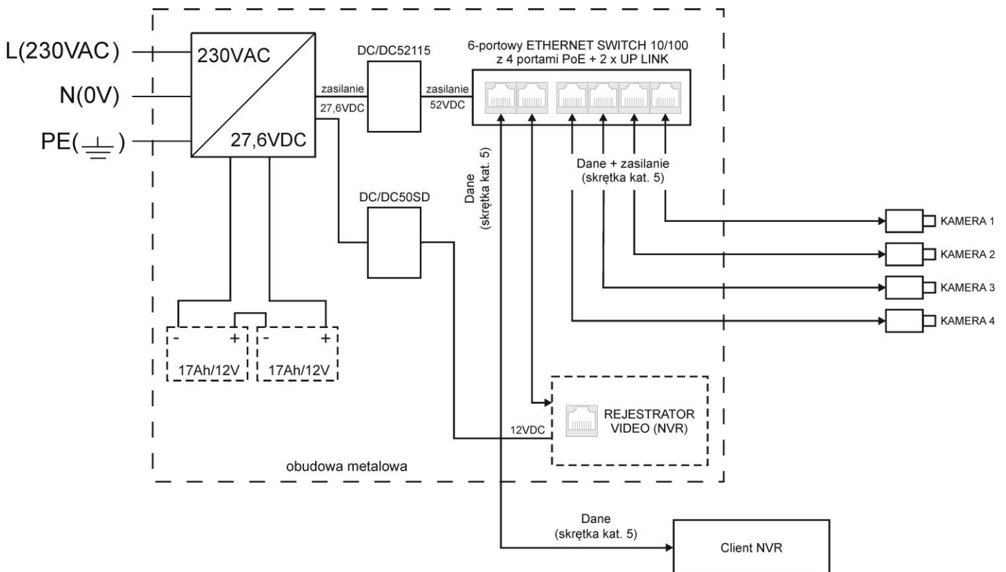
Rys. 1. Schemat blokowy.
