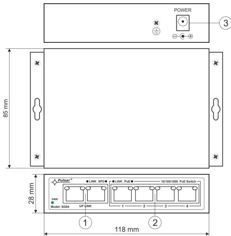
Rys. 3. Widok switch'a.
