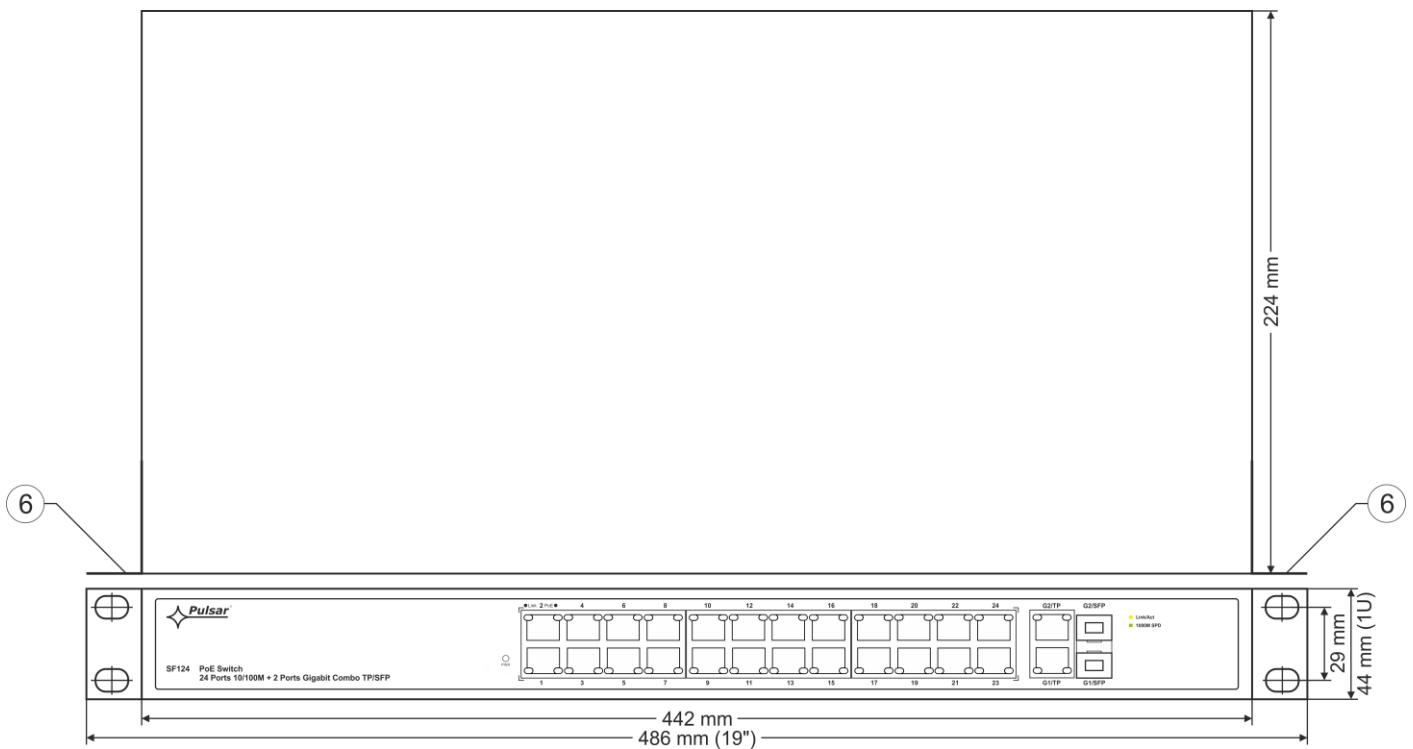
Rys. 4. Widok switch'a.
