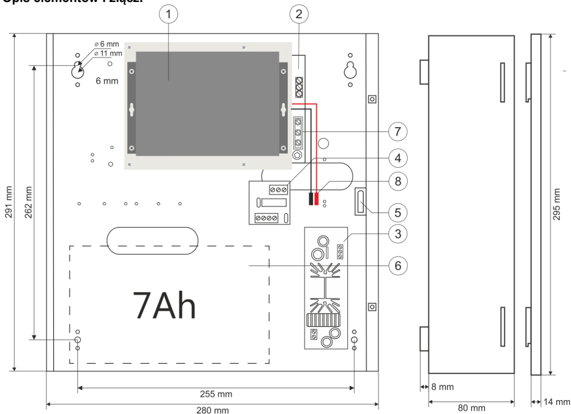
Rys. 2. Widok obudowy.
