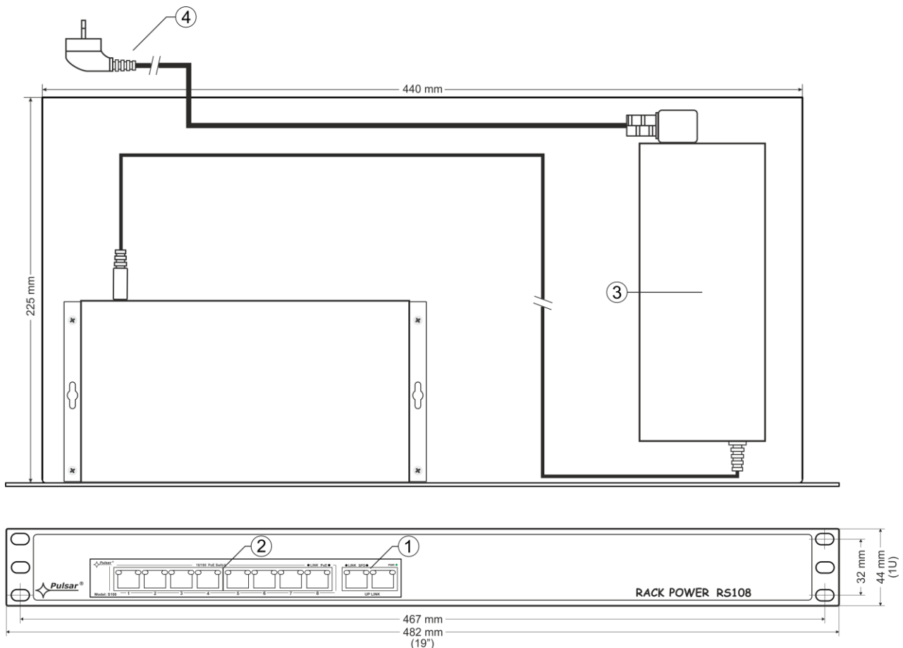
Rys. 2. Widok obudowy.
