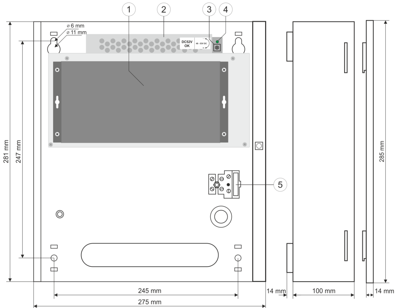
Rys. 2. Widok obudowy.
