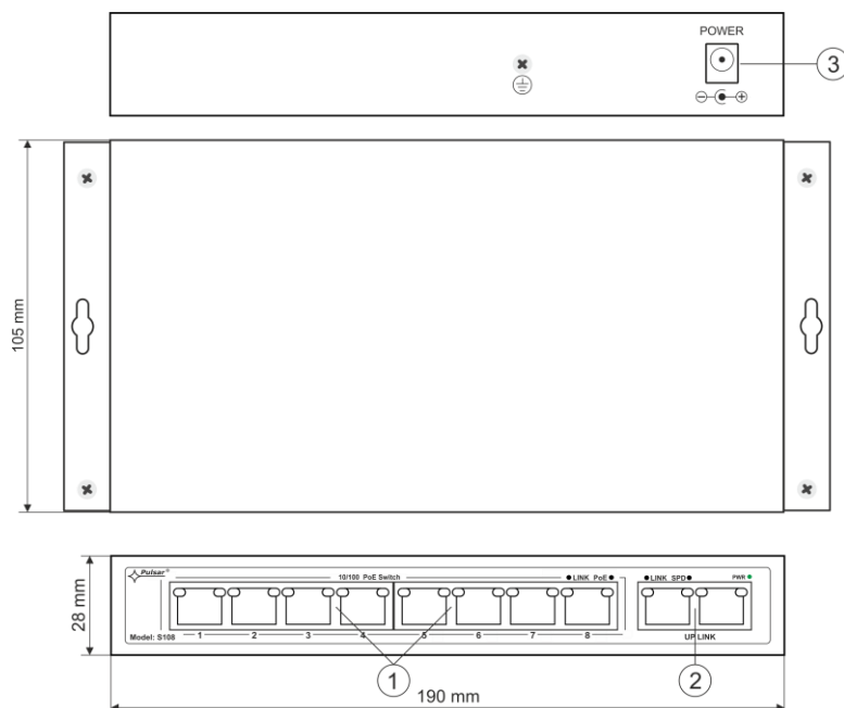
Rys. 3. Widok switch'a.
