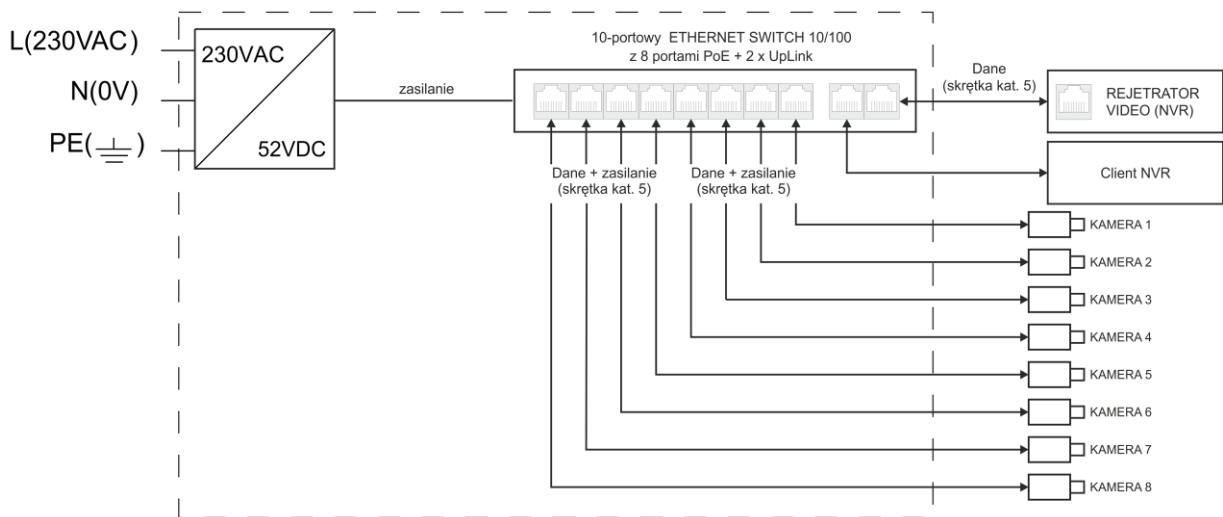
Rys. 1. Schemat blokowy.
