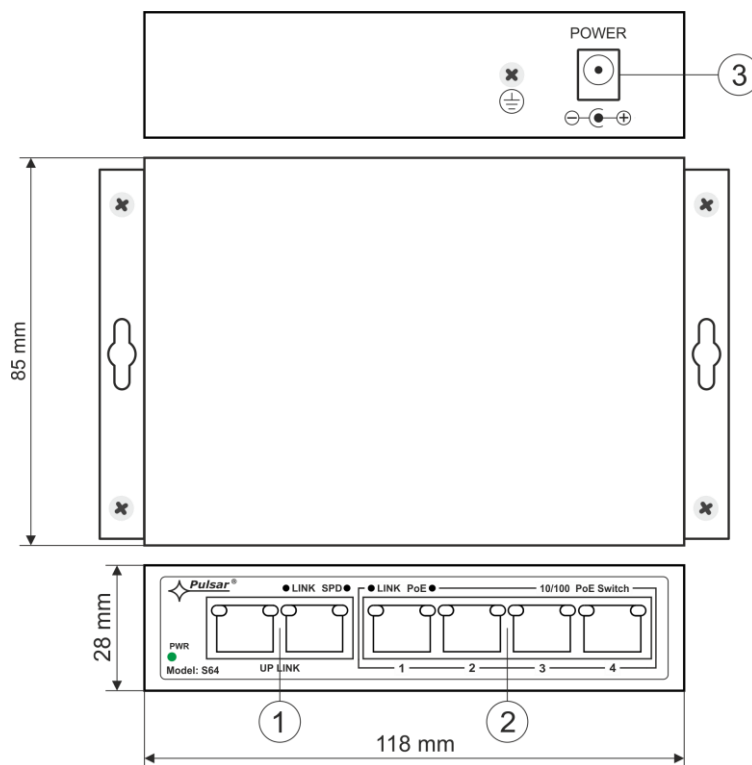
Rys. 3. Widok switch'a.
