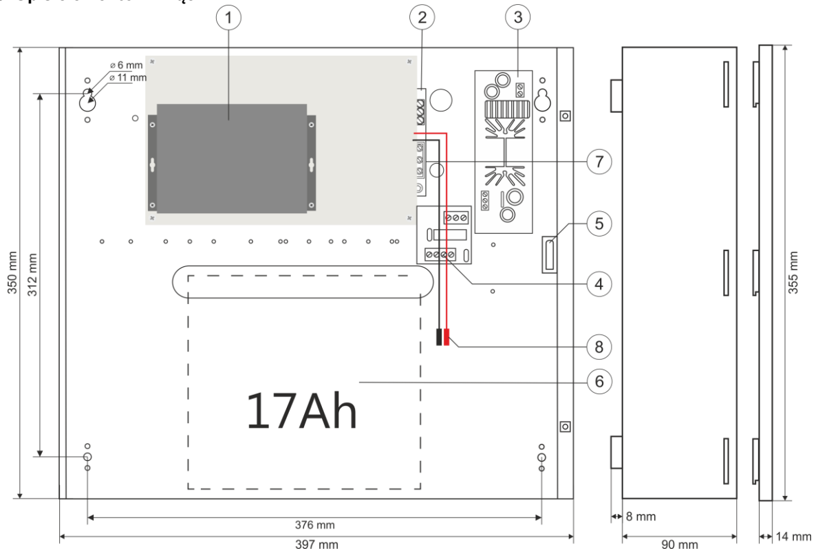
Rys. 2. Widok obudowy.
