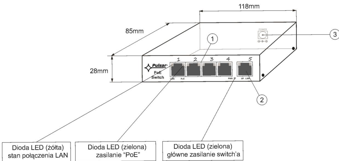
Rys. 3 Widok switch'a.
