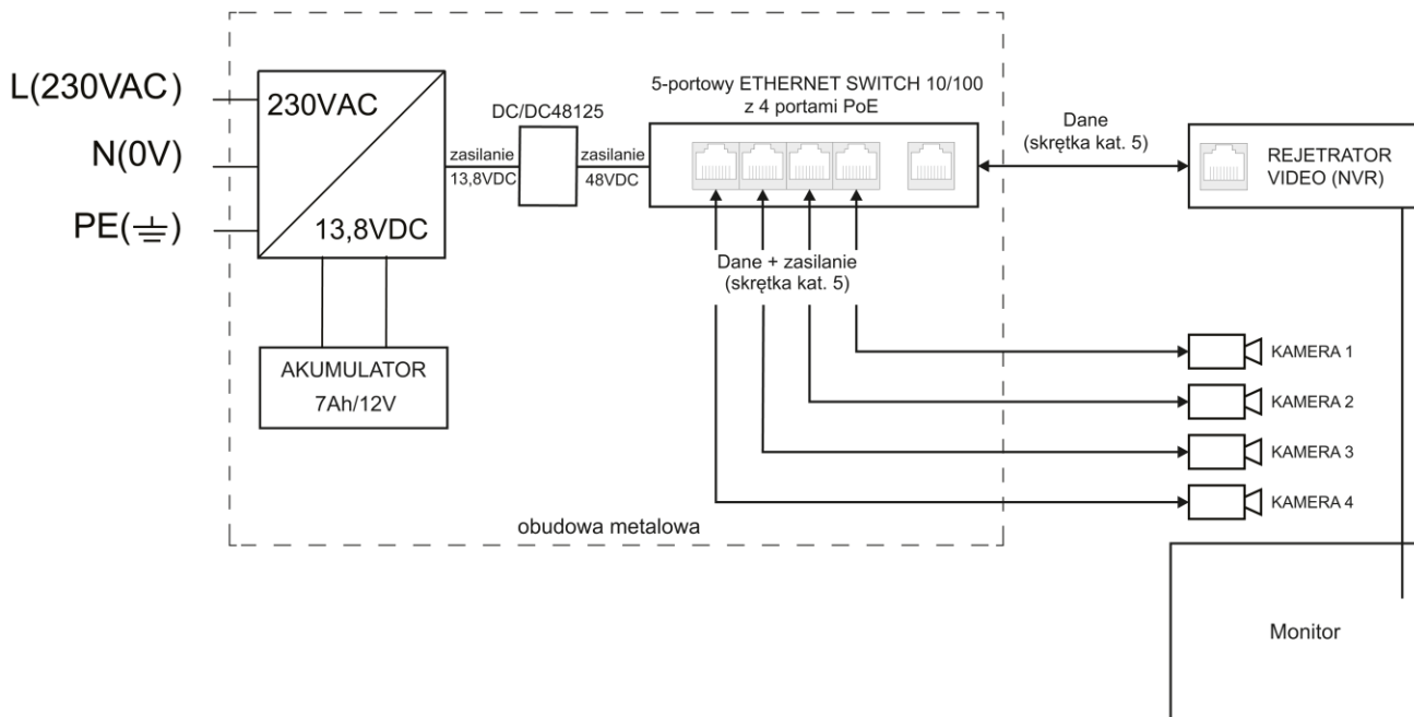
Rys 1. Schemat blokowy.
