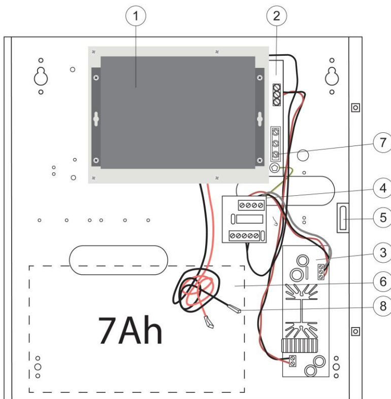
Rys. 2. Widok obudowy.
