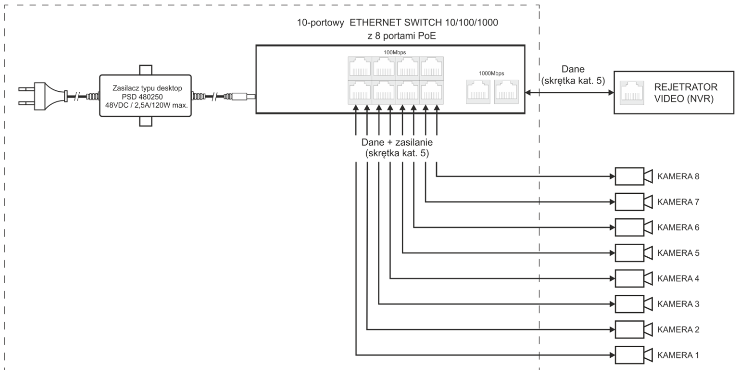
Rys. 1 Schemat blokowy.
