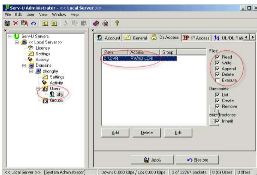
Rys. 5-15a. Ustawianie FTP.
