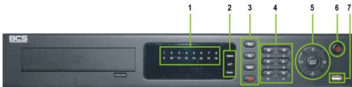
Rys. 2-1 Wygląd panela przedniego serii HF-L.
