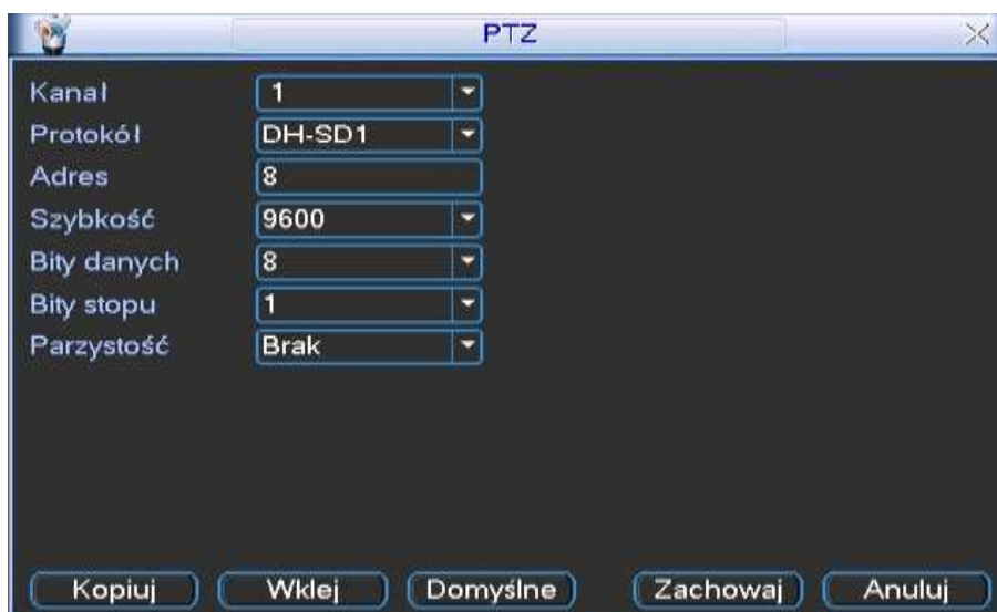
Rys. 5-18. Ustawianie PTZ.
