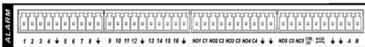
Rys. 3-6. Rozmieszczenia wejść / wyjść alarmowych rejestratora serii HF-L.
