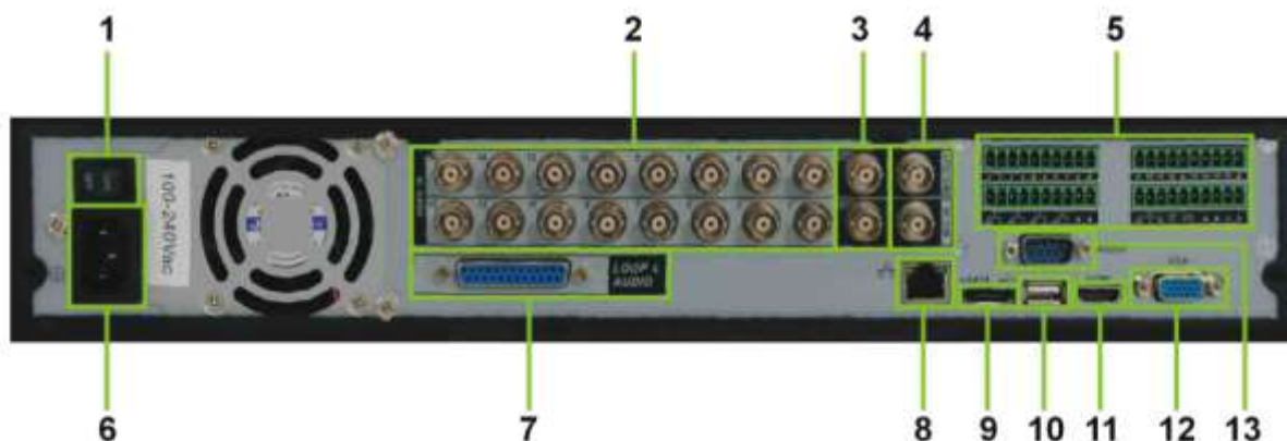
Rysunek 2-2. Wygląd panela tylnego rejestratora serii HF-L.
