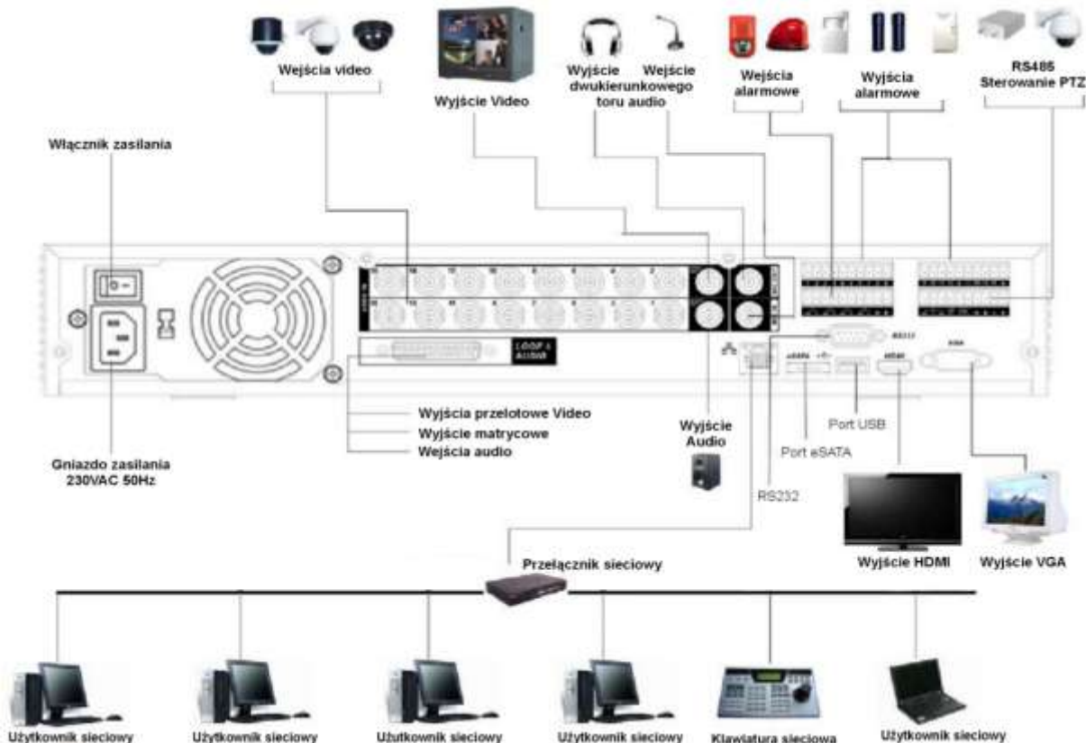
Rysunek 2-3. Przykładowy schemat podłączenia urządzeń peryferyjnych do rejestratora serii HF-L.
