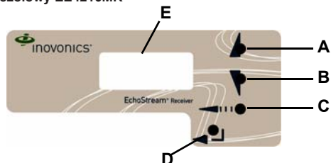
Rysunek 1. Panel czołowy odbiornika
