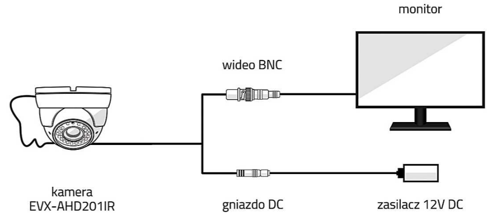
Sposób podłączenia
