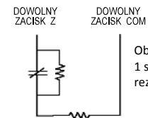
Rysunek 1-4 Podwójne rezystory końcowe
