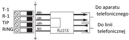
Rysunek 1-6 Podłączanie linii telefonicznej
