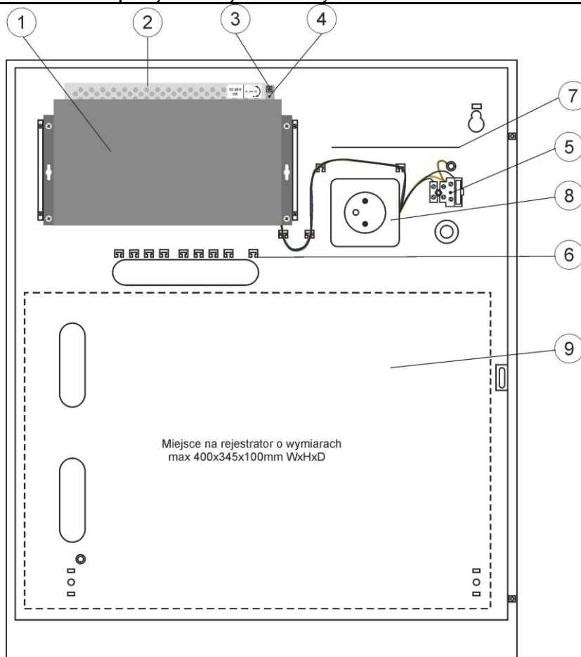
Rys.2. Widok obudowy.
