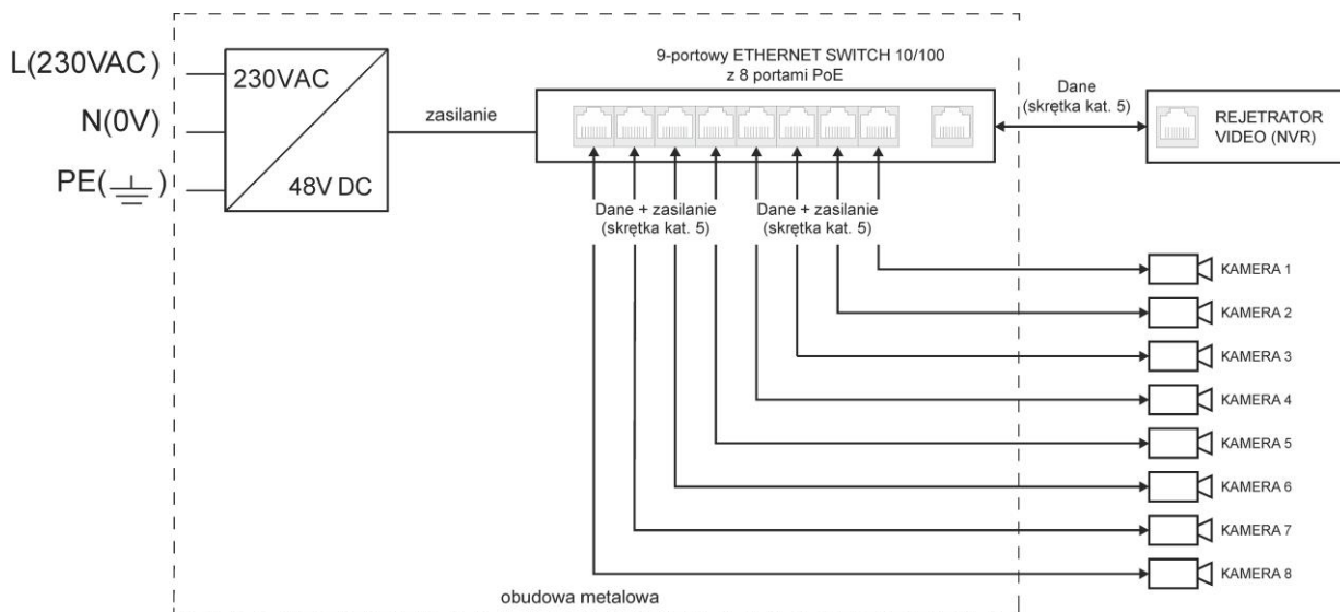
Rys. 1 Schemat blokowy.
