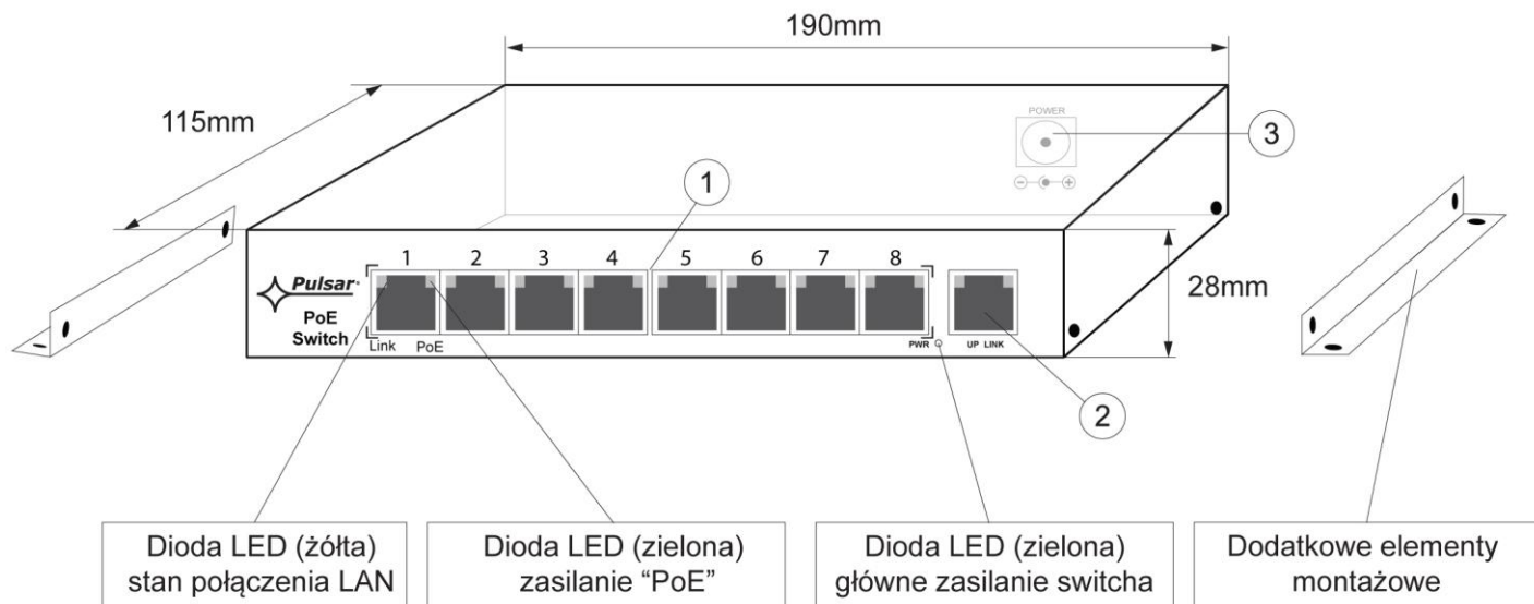
Rys. 3 Widok switch'a.
