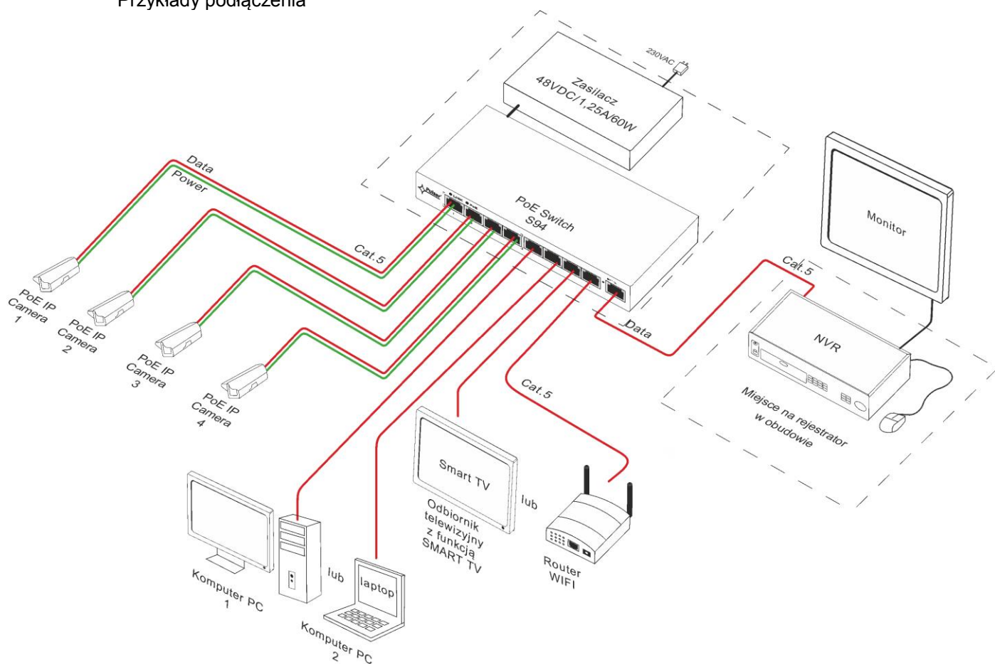
Przykłady podłączenia
