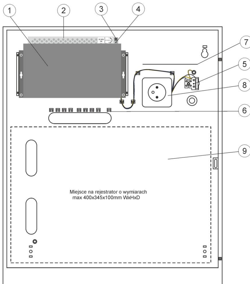
Rys.2 Widok obudowy.
