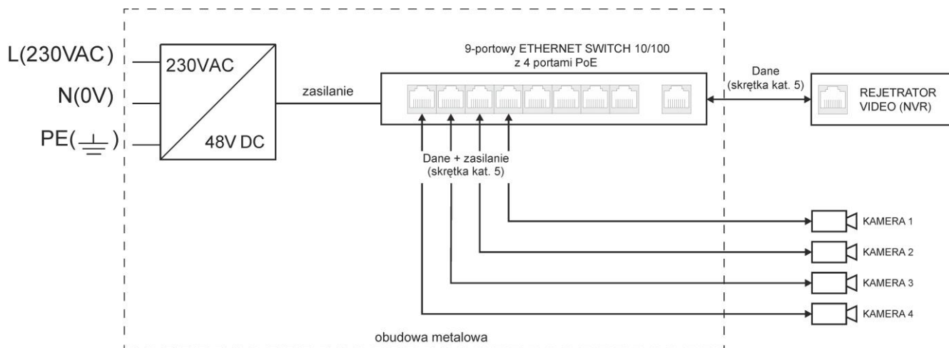
Rys. 1 Schemat blokowy.
