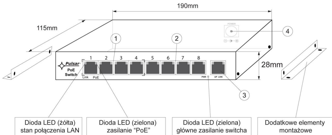
Rys. 3 Widok switch'a.
