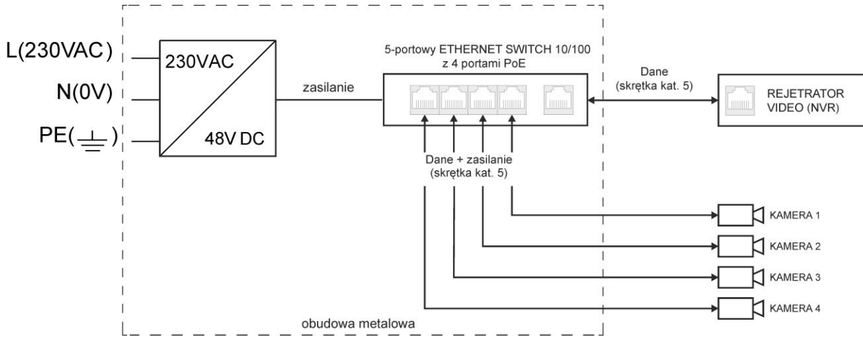
Rys. 1 Schemat blokowy.
