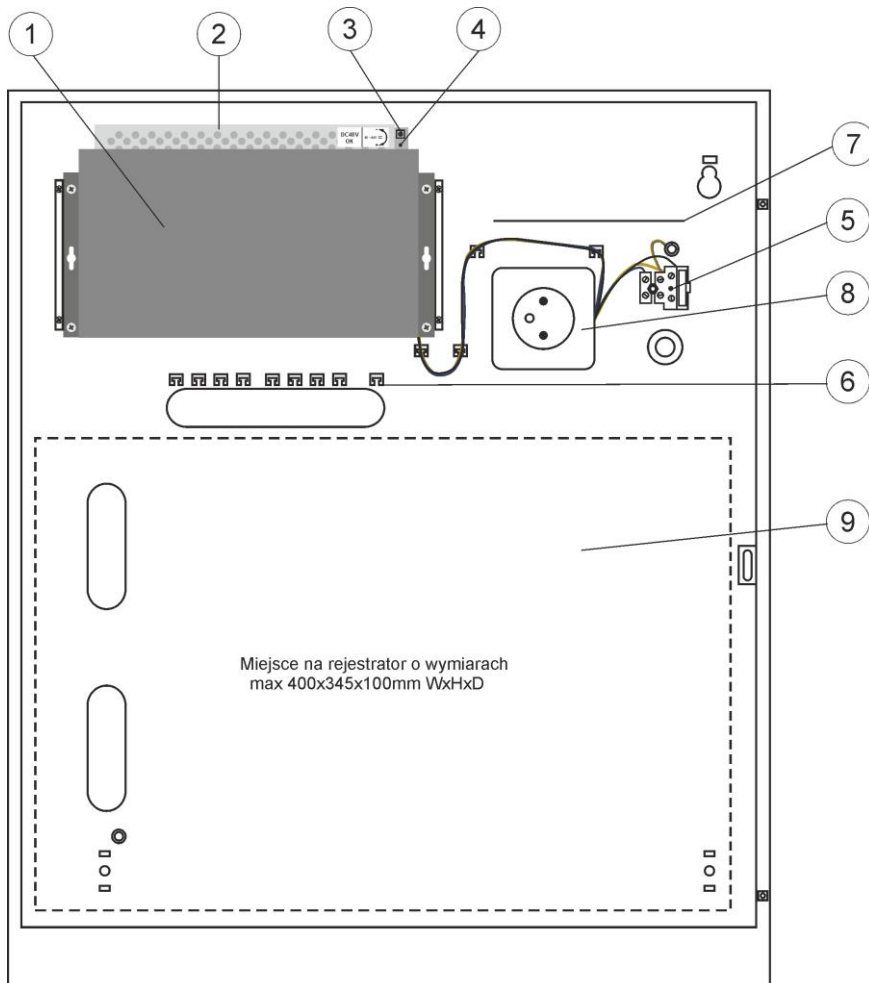
Rys. 2 Widok obudowy.
