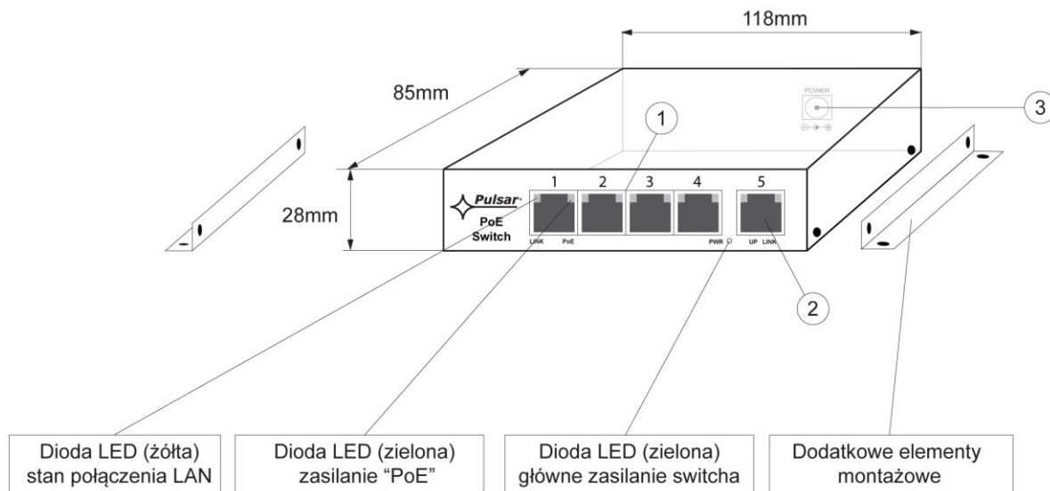
Rys. 3 Widok switch'a.
