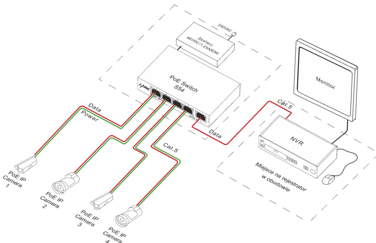
Przykłady podłączenia
