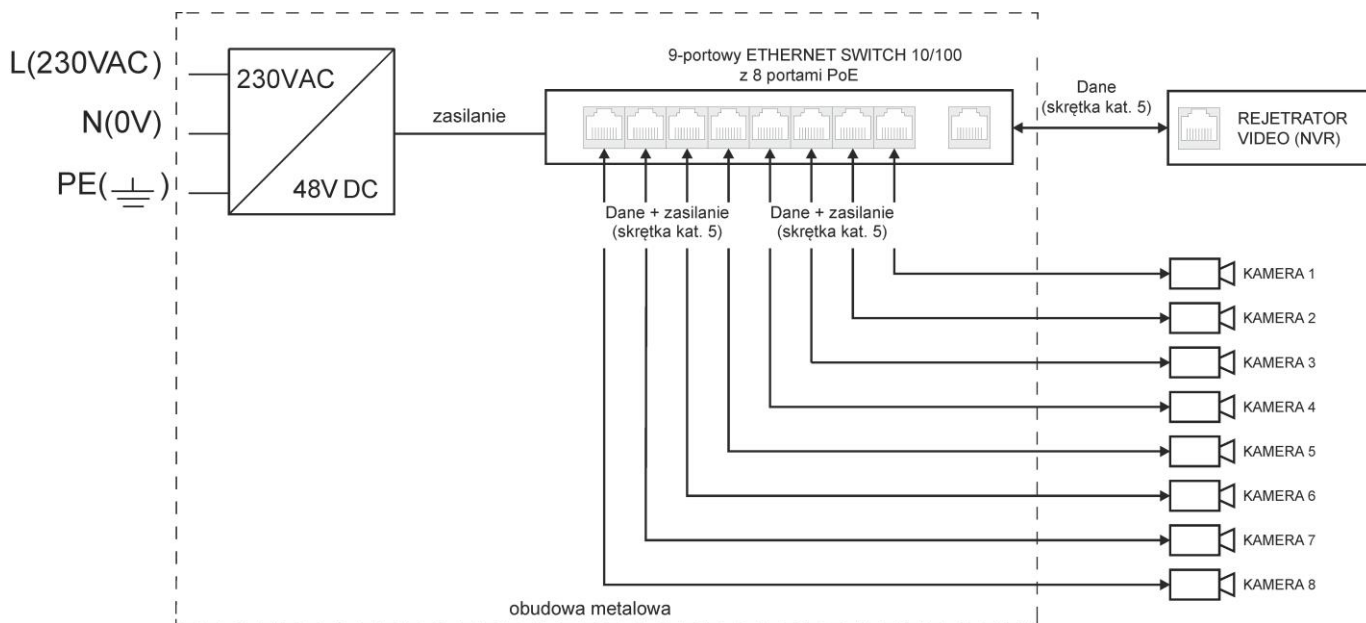
Rys. 1 Schemat blokowy.
