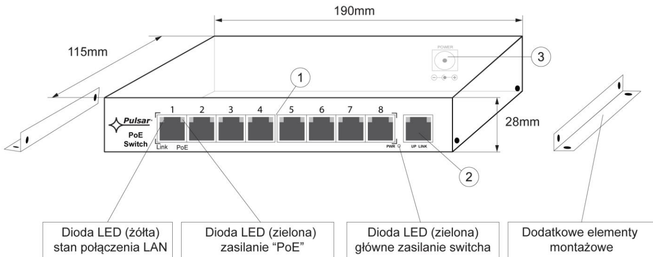
Rys. 3 Widok switch'a.
