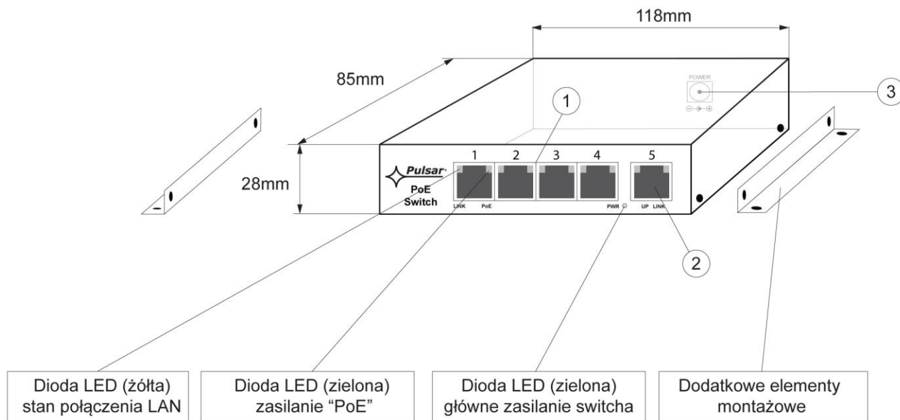
Rys. 3 Widok switch'a.
