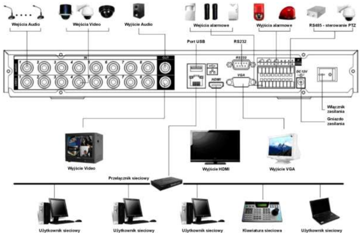
Rysunek 2-5a. Przykładowy schemat podłączenia urządzeń peryferyjnych do rejestratora 8-kanalowego serii HF-A.
