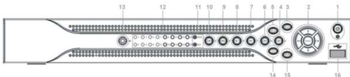
Rys. 2-1 Wygląd panela przedniego rejestratora serii HF-A.
