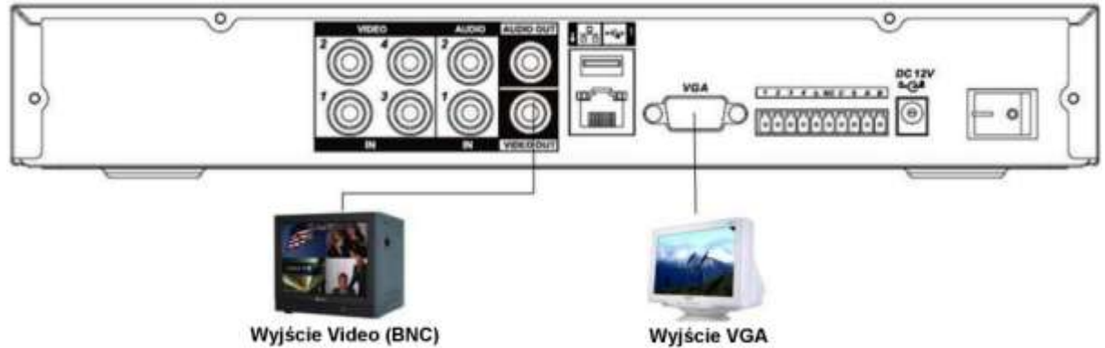
Rys. 3-2b Podłączenie monitorów do rejestratora HE-AS (HE-AN).
