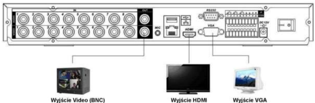
Rys. 3-2a. Podłączenie monitorów do rejestratora HF-A.
