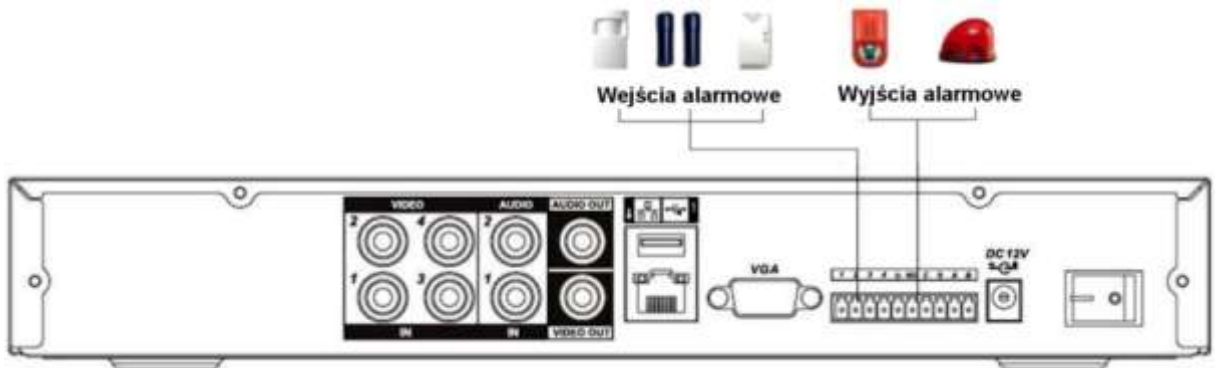
Rys. 3-4b. Podłączenie wejść i wyjść alarmowych w rejestratorach. serii HE-AS.
