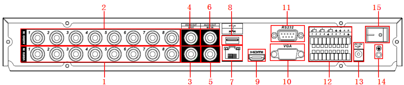
Rysunek 2-2a. Wygląd tylnego panelu rejestratora 4/8 kanałowego serii HF-A.
