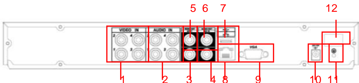
Rysunek 2-4. Wygląd tylnego panelu rejestratora 4-kanalowego serii HE-AN.
