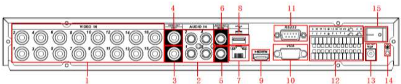
Rysunek 2-2c. Wygląd tylnego panelu rejestratora 16-kanałowego serii HF-A.
