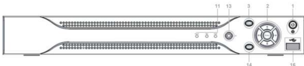
Rys. 2-1a Wygląd panela przedniego rejestratora serii HE-AS oraz HE-AN.
