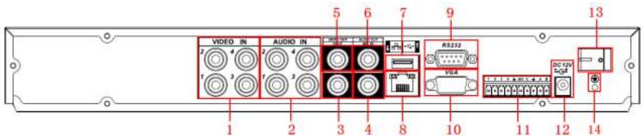
Rysunek 2-3a. Wygląd tylnego panelu rejestratora 4-kanalowego serii HE-AS.
