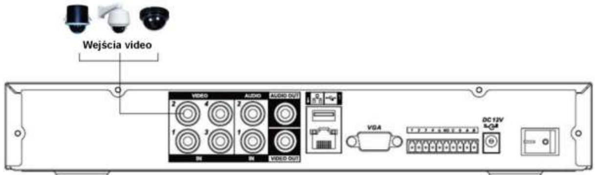
Rys. 3-1b. Przykładowe podłączenie kamer do rejestratora serii HE-AS (HE-AN).
