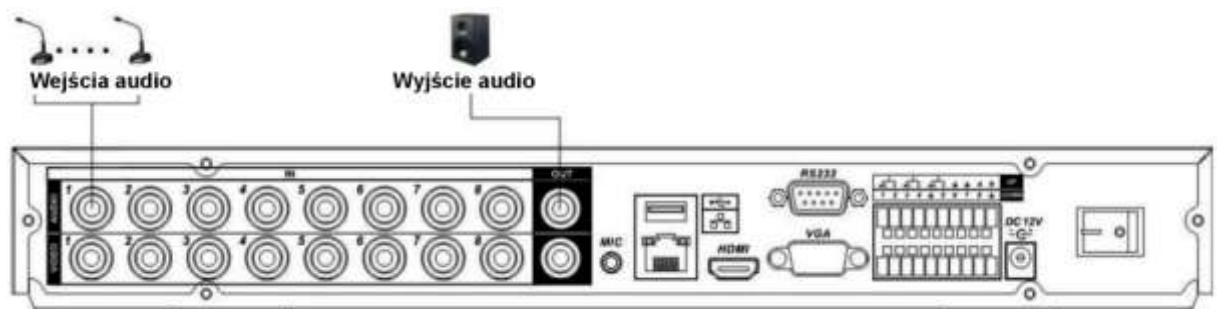
Rys. 3-3a. Podłączenia wejść i wyjść audio do rejestratora 8-kanalowego z serii HF-A.
