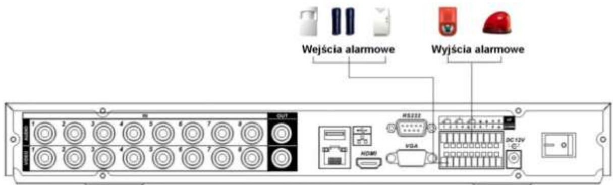
Rys. 3-4a. Podłączenie wejść i wyjść alarmowych w rejestratorach. serii HF-A.
