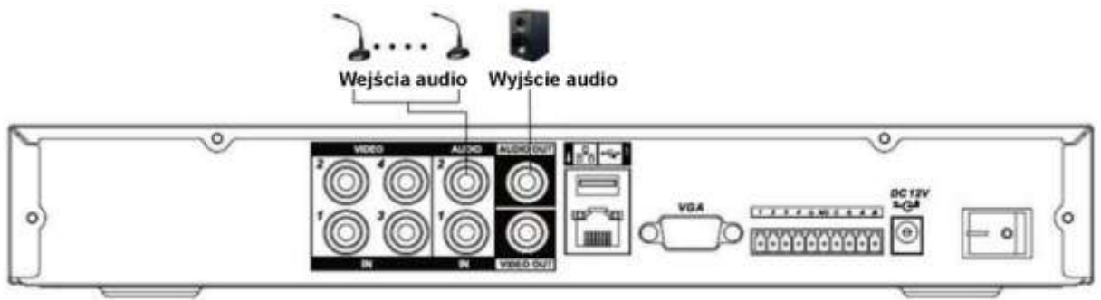
Rys. 3-3b. Podłączenia wejść i wyjść audio do rejestratora 4-kanalowego z serii HE-AS (HE-AN).
