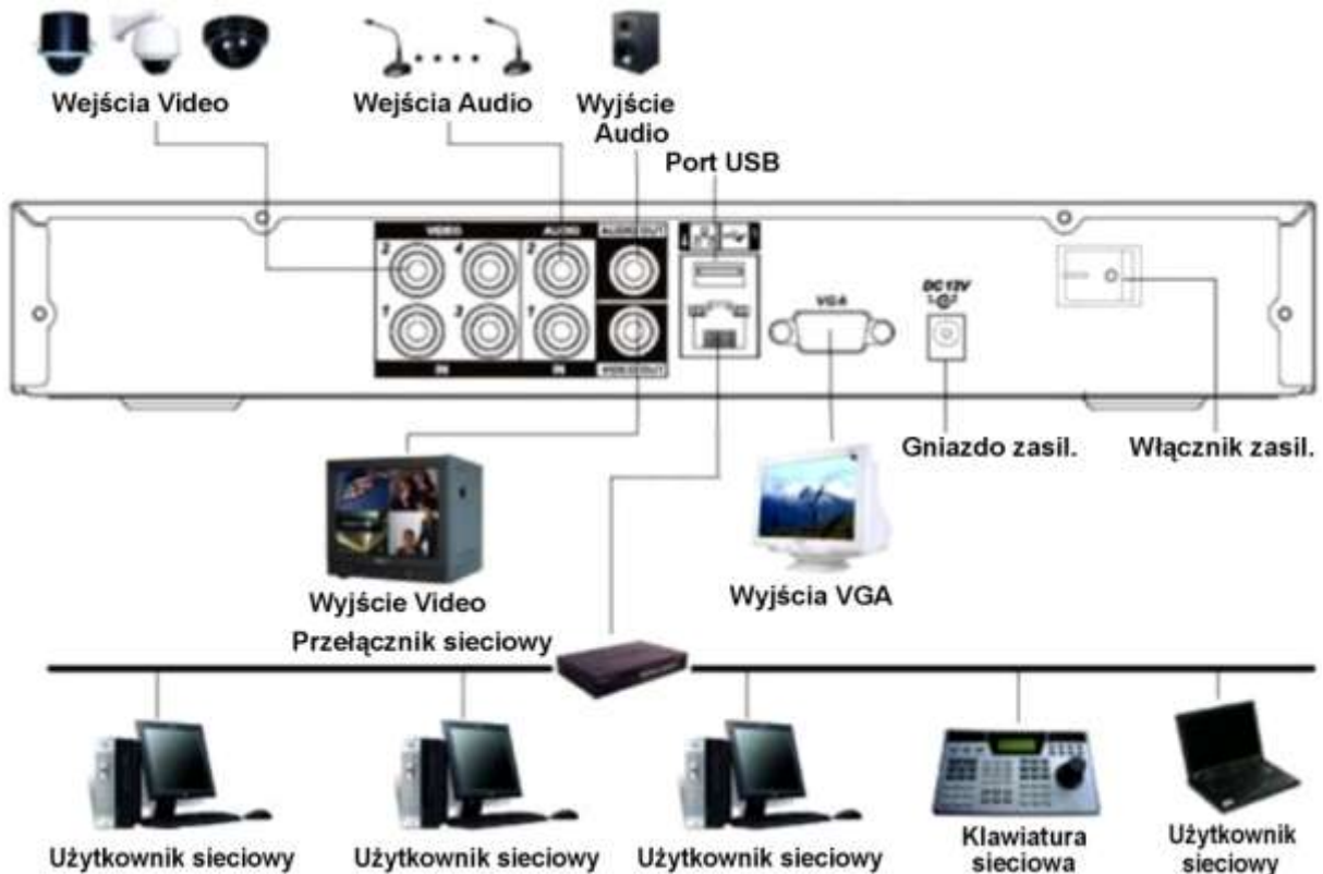
Rysunek 2-5c. Przykładowy schemat podłączenia urządzeń peryferyjnych do rejestratora 4-kanalowego serii HE-AN.
