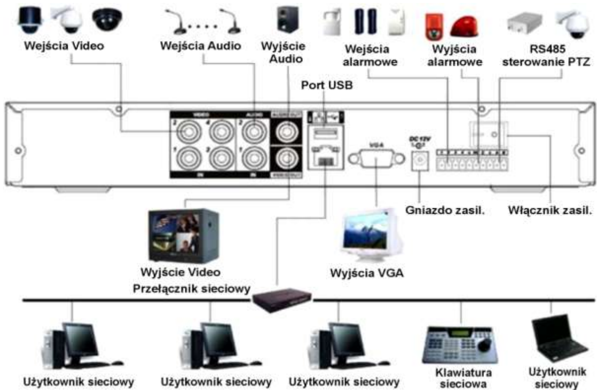
Rysunek 2-5b. Przykładowy schemat podłączenia urządzeń peryferyjnych do rejestratora 4-kanalowego serii HE-AS.
