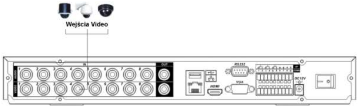
Rys. 3-1a. Przykładowe podłączenie kamer do rejestratora serii HF-A.
