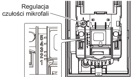
Schemat ustawień zasięgu detekcji
