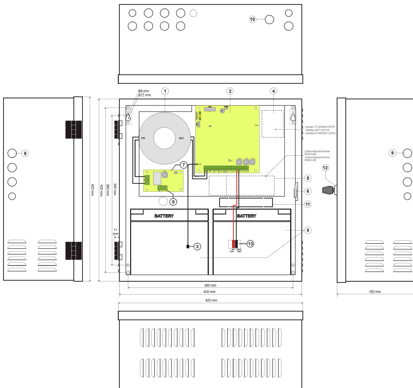
Rys.4. Widok zasilacza.
