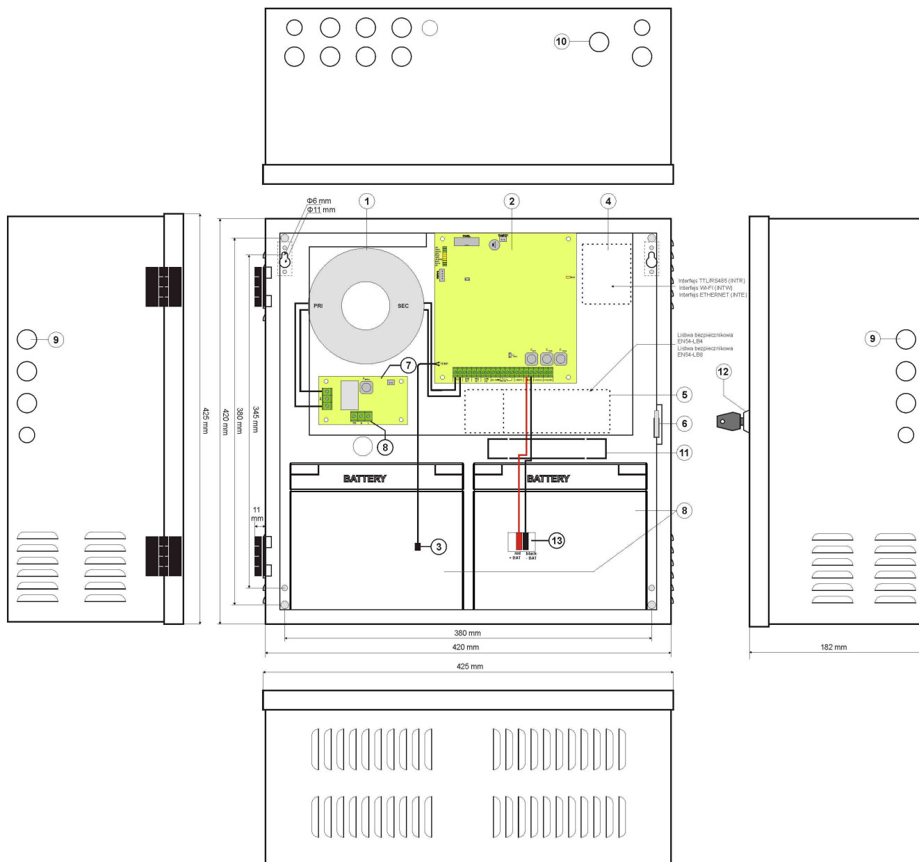
Rys.4. Widok zasilacza.
