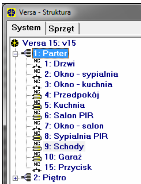
Rys. 6. Lista stref i wejść w formie drzewka w zakładce „System” w oknie „Versa – Struktura” (przykładowa konfiguracja).
