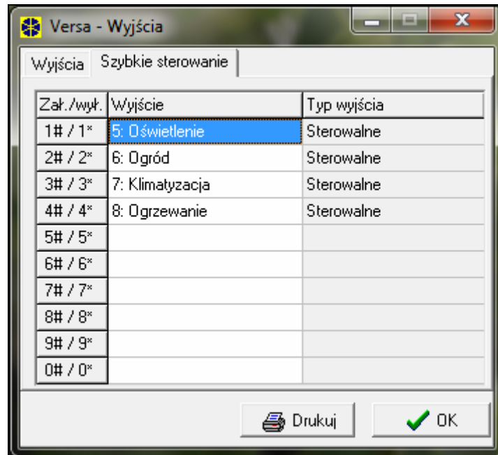
Rys. 11. Przypisywanie wyjść do odpowiednich klawiszy manipulatora w programie DLOADX (przykładowa konfiguracja).
