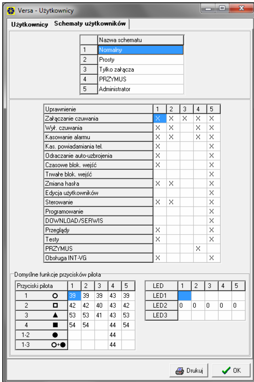
Rys. 19. Programowanie schematów użytkowników w oknie „Versa – Użytkownicy” w programie DLOADX (przykładowe ustawienia).
