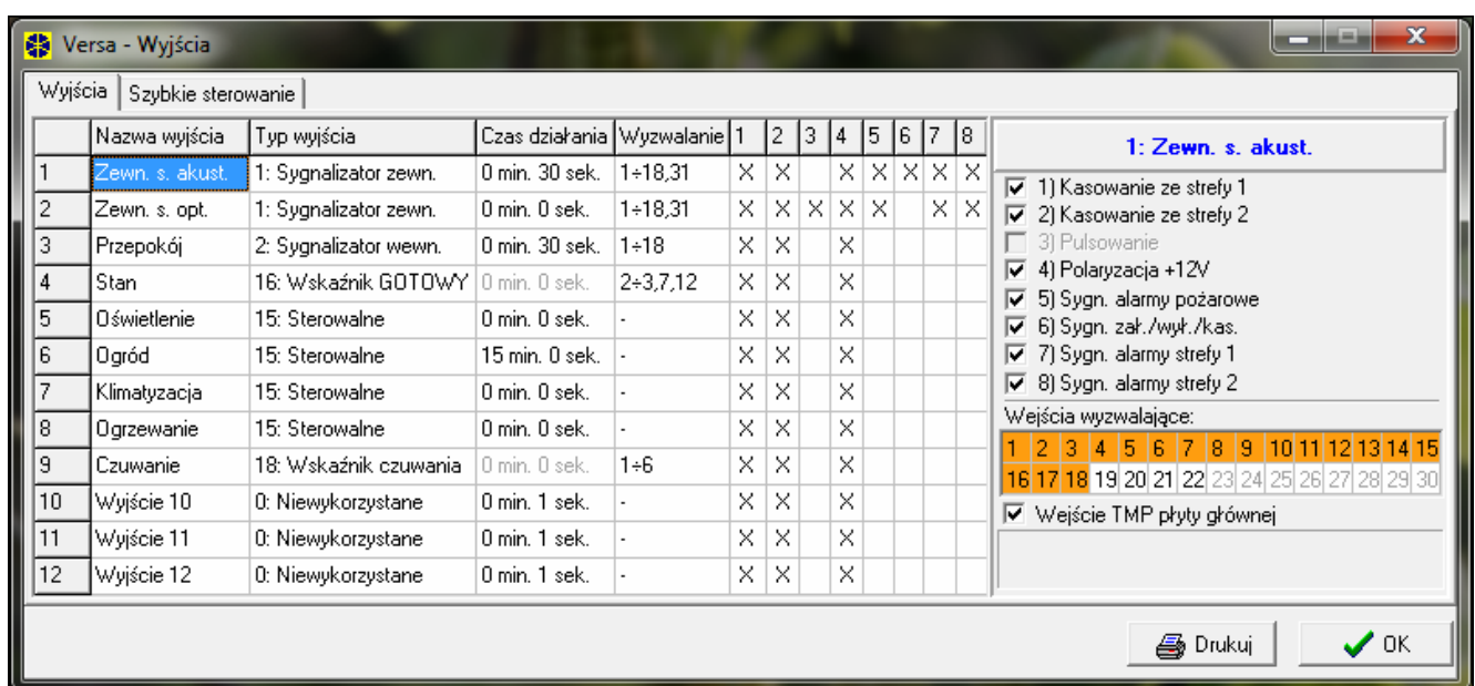
Rys. 10. Okno „Versa – Wyjścia” w programie DLOADX.
