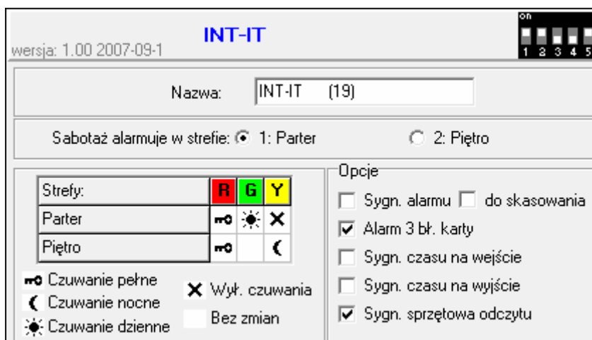
Rys. 15. Programowanie ustawień modułu sterowania strefami w programie DLOADX (przykładowa konfiguracja).
