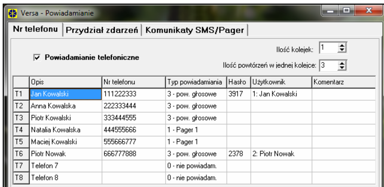
Rys. 18. Programowanie parametrów powiadamiania w programie DLOADX (przykładowa konfiguracja).
