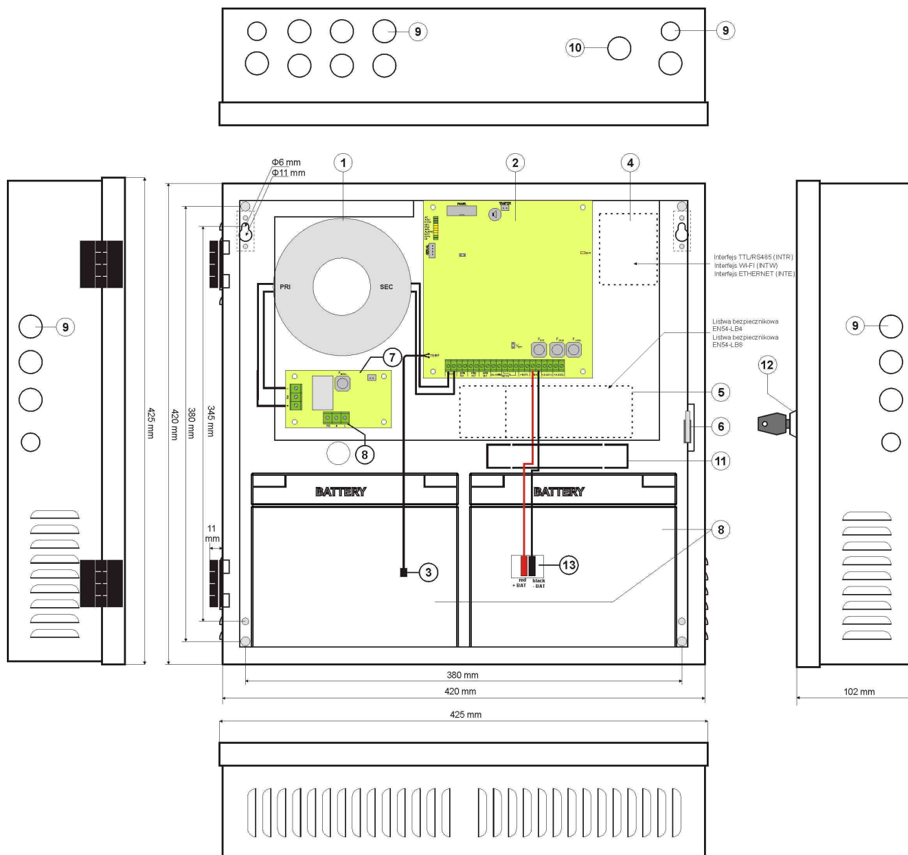
Rys.4. Widok zasilacza.
