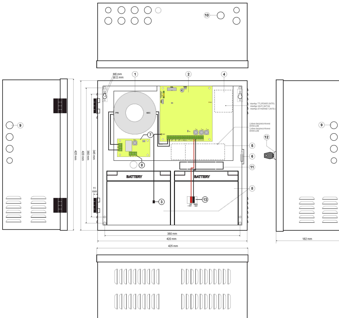
Rys.4. Widok zasilacza.
