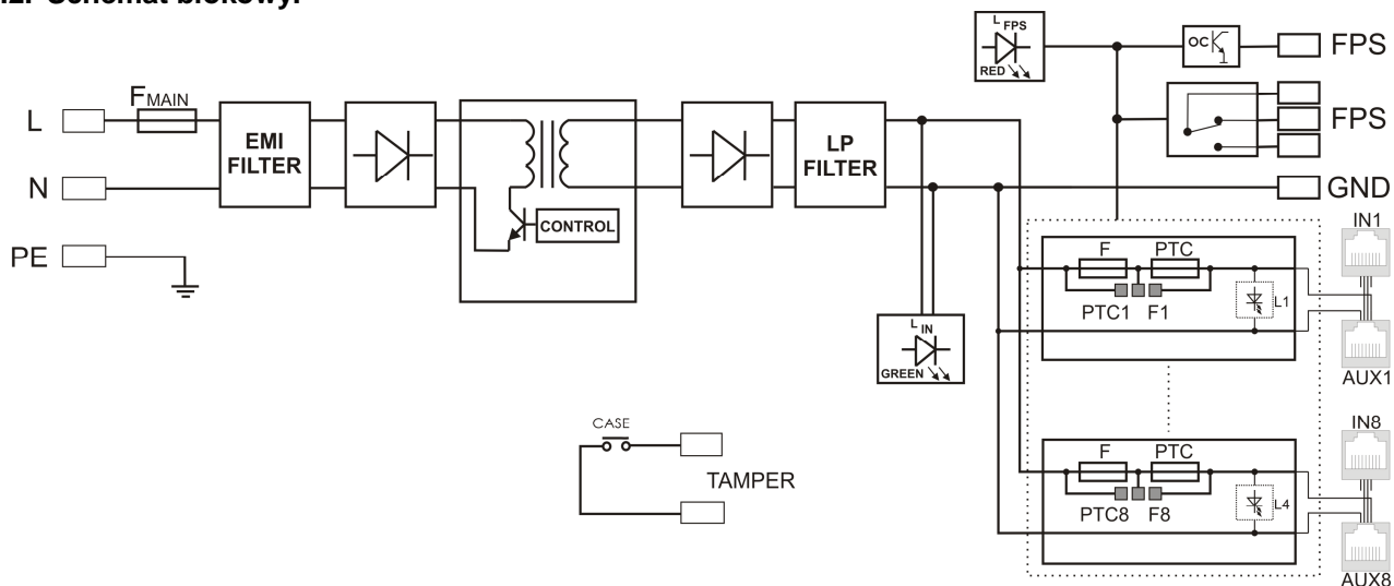
Rys. 1. Schemat blokowy zasilacza.
