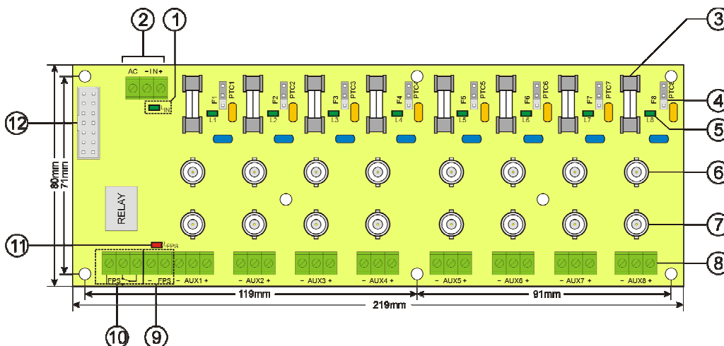
Rys. 2. Rozmieszczenie elementów.
