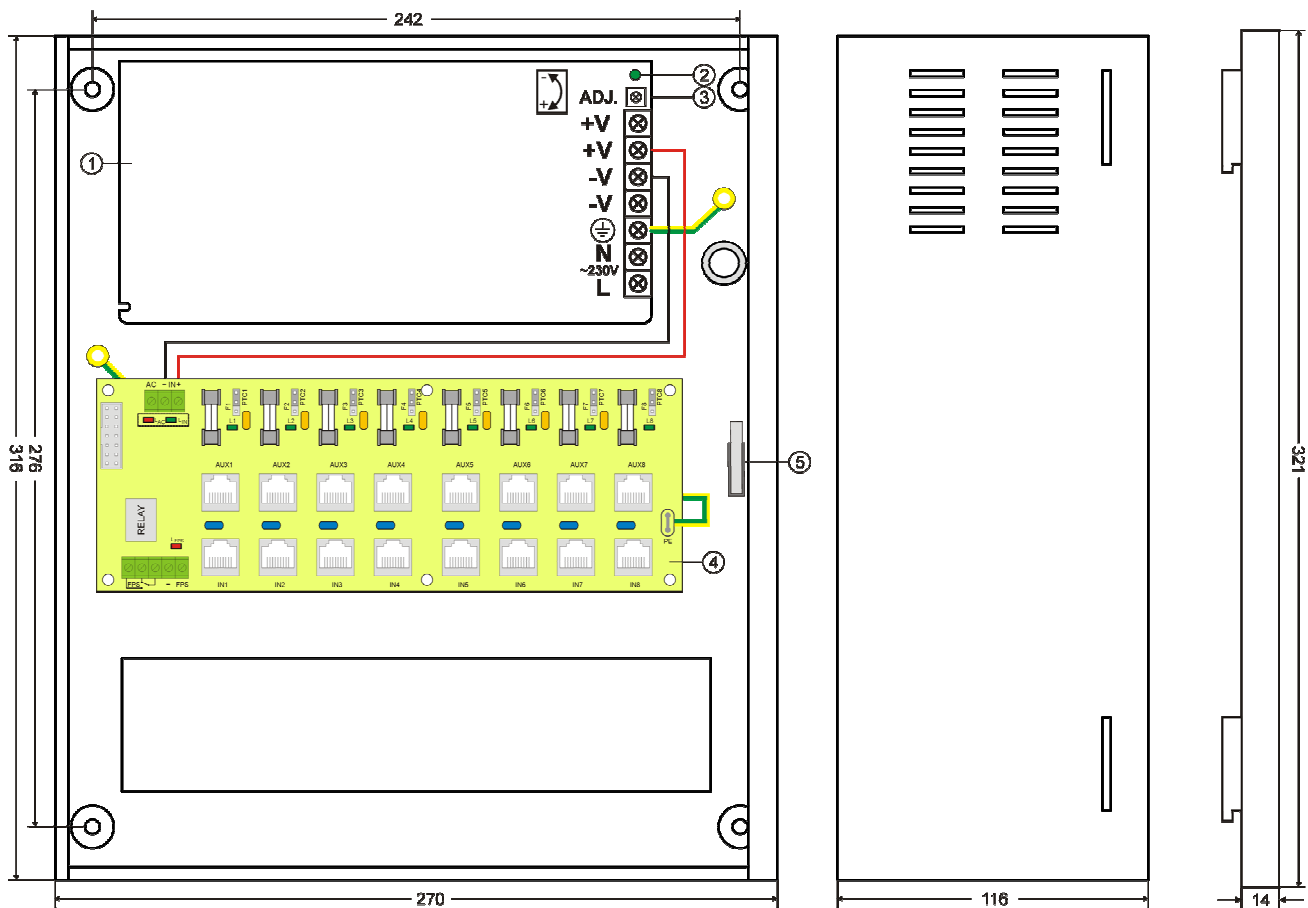
Rys. 3. Widok zasilacza.
