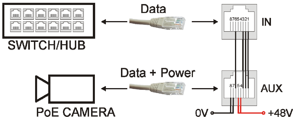
Rys. 4. Opis pinów złącz IN oraz AUX.
