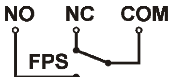
Rys. 6. Schemat elektryczny wyjścia przekaźnikowego
