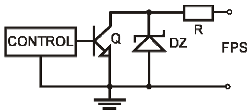
Rys. 5. Schemat elektryczny wyjścia OC.
