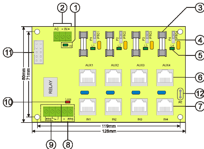
Rys. 2. Rozmieszczenie elementów.
