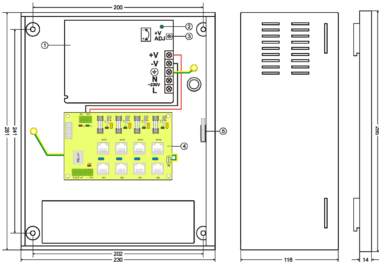
Rys. 3. Widok zasilacza.
