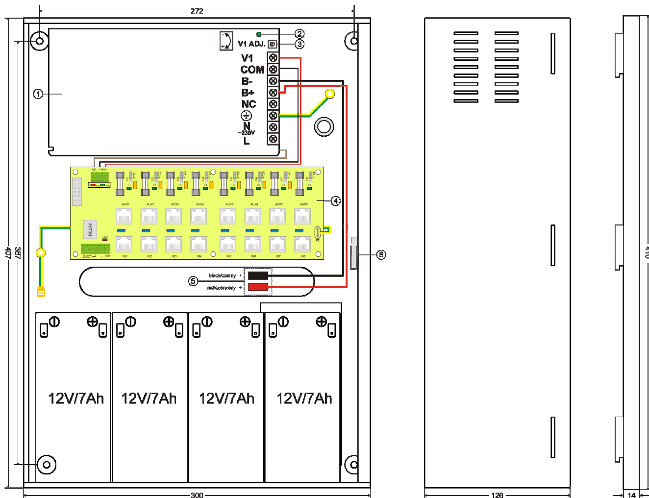
Rys. 3. Widok zasilacza.
