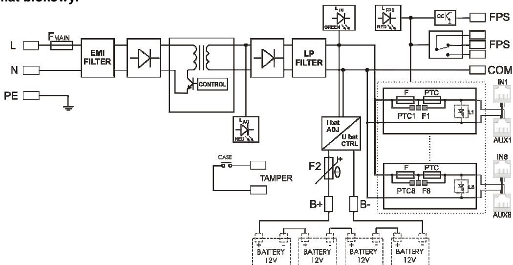
Rys. 1. Schemat blokowy zasilacza.
