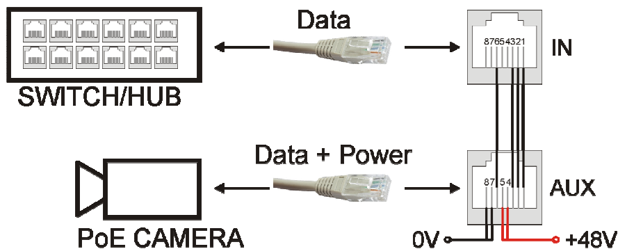
Rys. 4. Opis pinów złącz IN oraz AUX.
