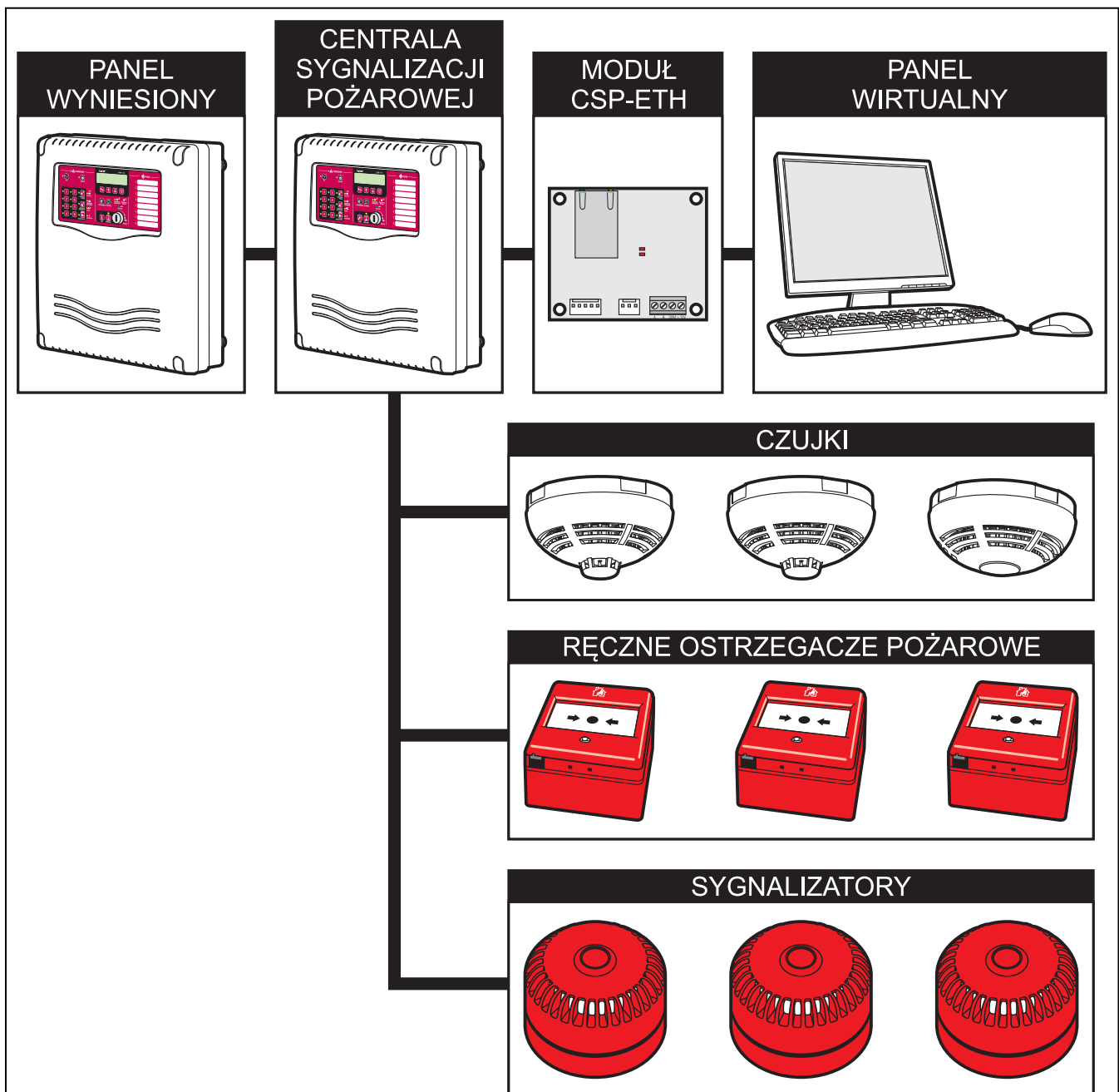
Rys. 1. Przykładowe elementy wchodzące w skład systemu sygnalizacji pożarowej.
