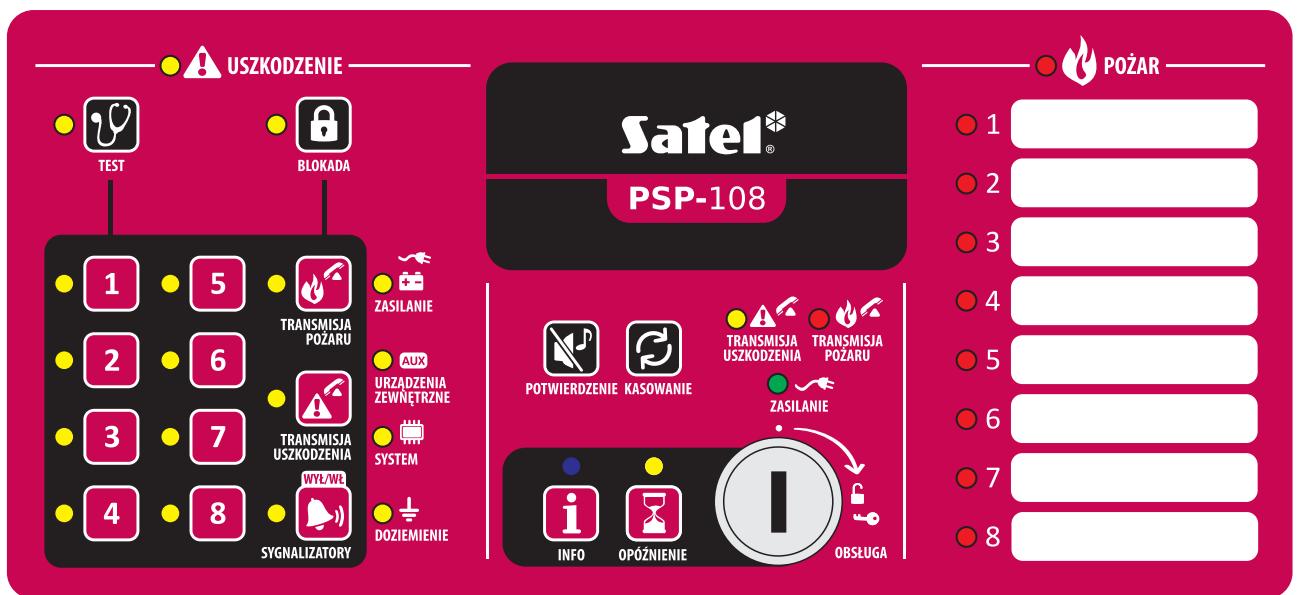
Rys. 7. Panel czołowy panelu wyniesionego PSP-108.
