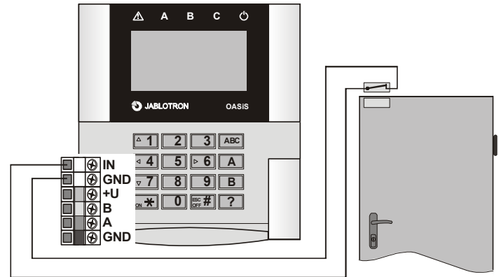
Schemat 2. Przykładowe podłączenia czujki przewodowej
