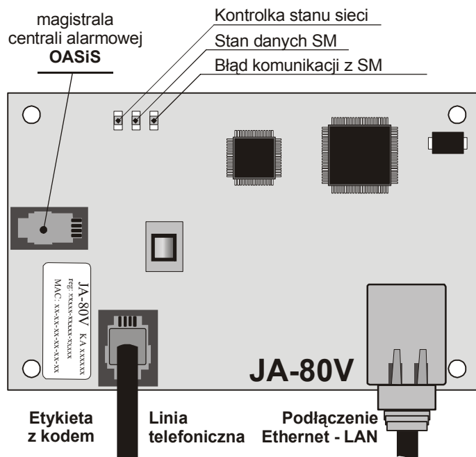
Rys.1 Podłączenie dialera
