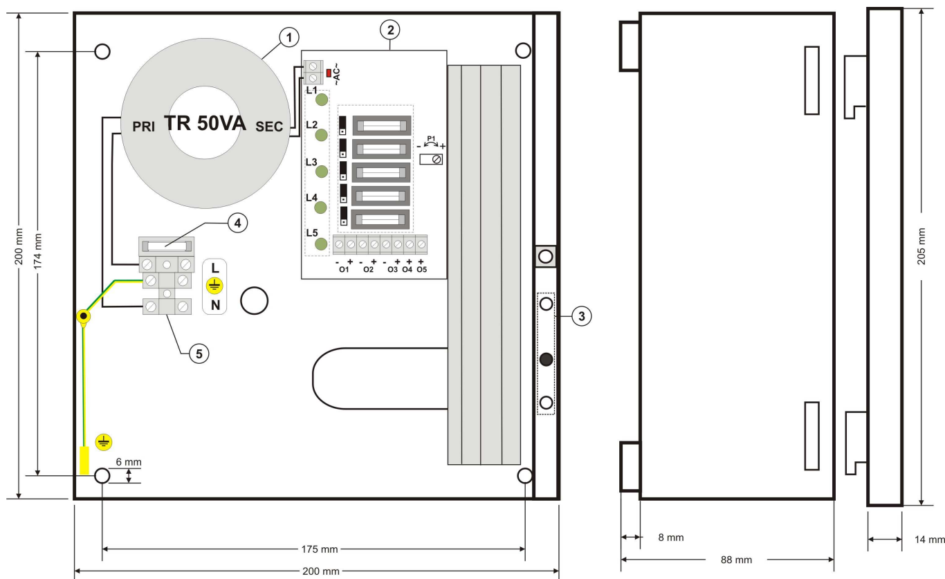
Rys.3. Widok zasilacza.
