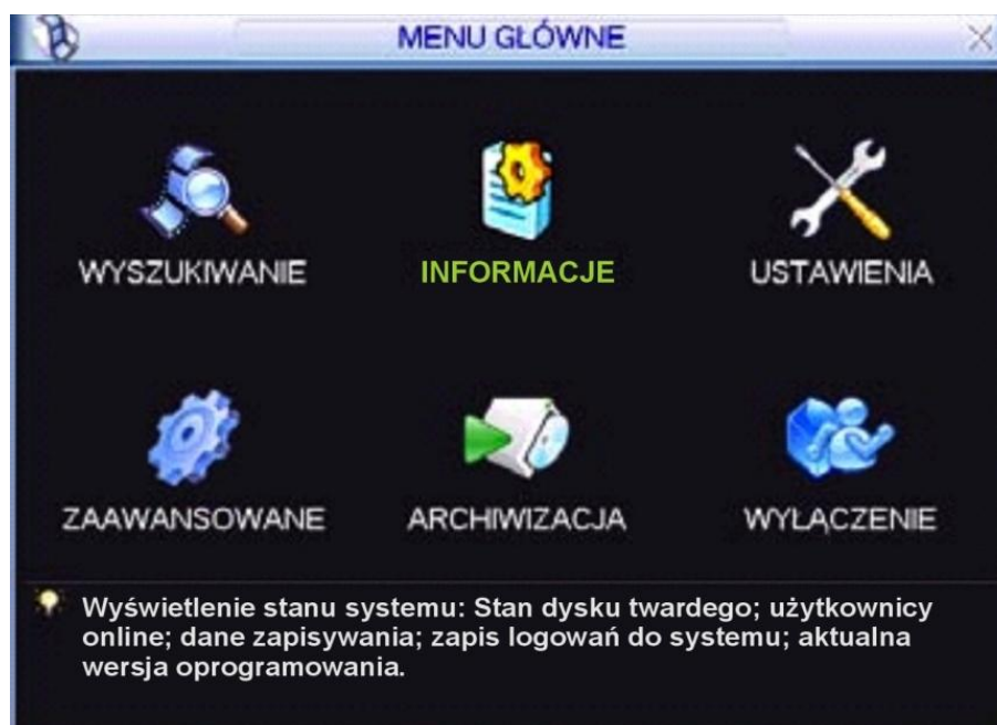
Rys. 4-2. Menu główne.
