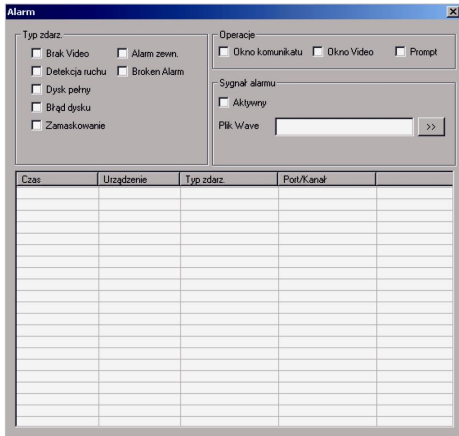
Rys. 7-61. Interfejs Alarm.
