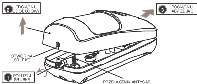
Rys. 3. Zdjęcie pokrywy
