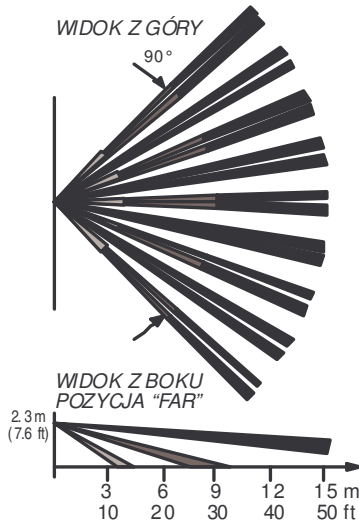
Rys. 2. Obszar chroniony
