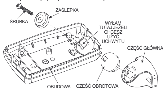
Rys. 6. Montaż uchwytu
