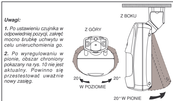
Rys. 8. Limity obrotu/pochylenia
