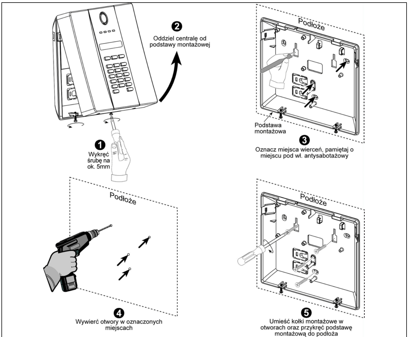
Rys. 3.1 – Montaż tylnej części obudowy
