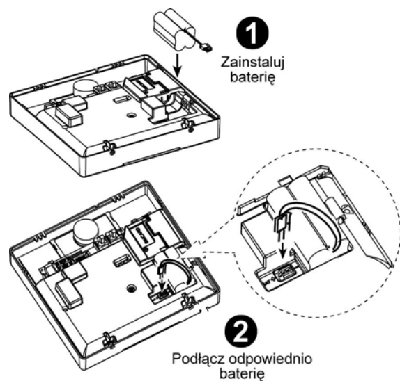
Rys. 3.3 – Instalacja baterii
