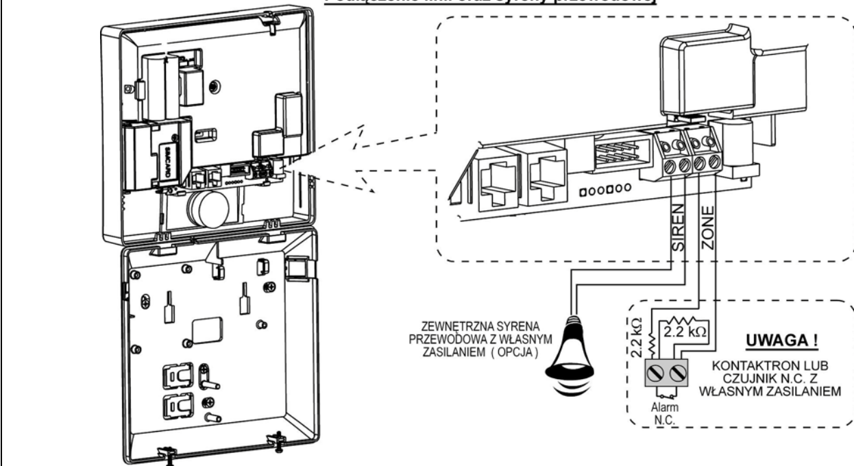
Rys. 3.2 - Okablowanie
