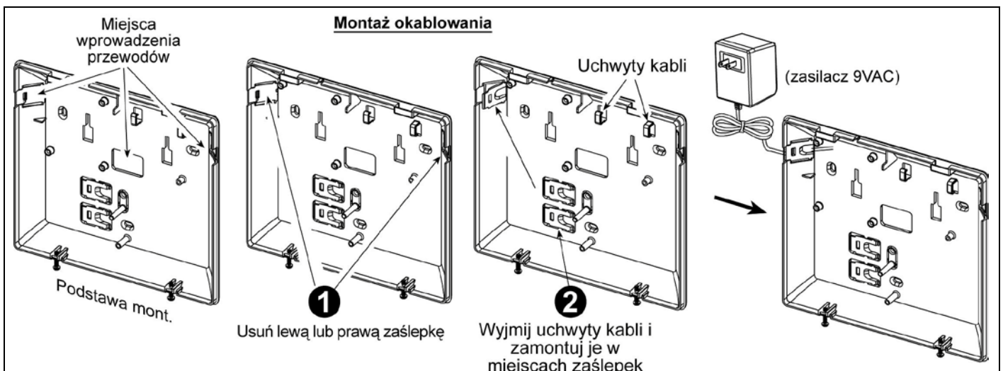
Rys. 3.1 – Montaż tylnej części obudowy
