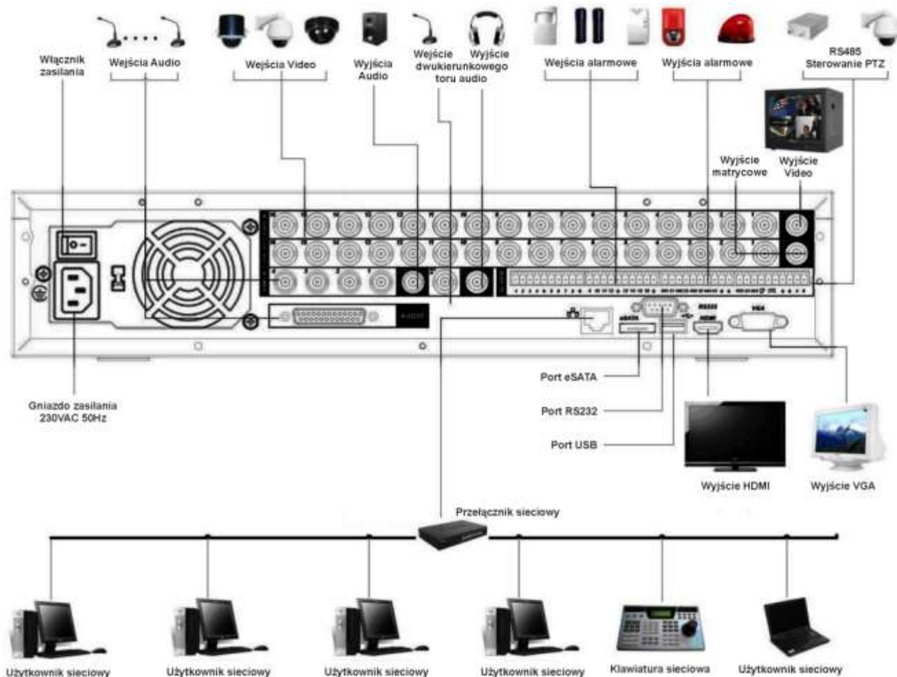
Rysunek 2-3. Przykładowy schemat podłączenia urządzeń peryferyjnych do rejestratora serii HF-S.
