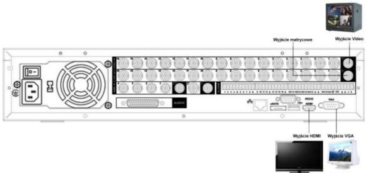
Rys. 3-2. Podłączenie monitorów do rejestratora.
