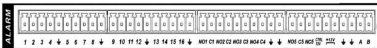
Rys. 3-6. Rozmieszczenia wejść / wyjść alarmowych rejestratora serii HF-S.
