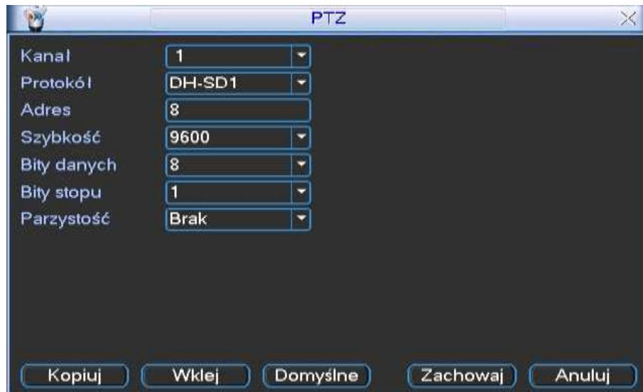
Rys. 5-18. Ustawianie PTZ.
