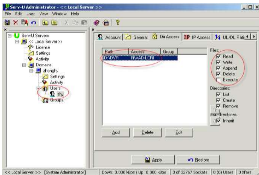
Rys. 5-15a. Ustawianie FTP.
