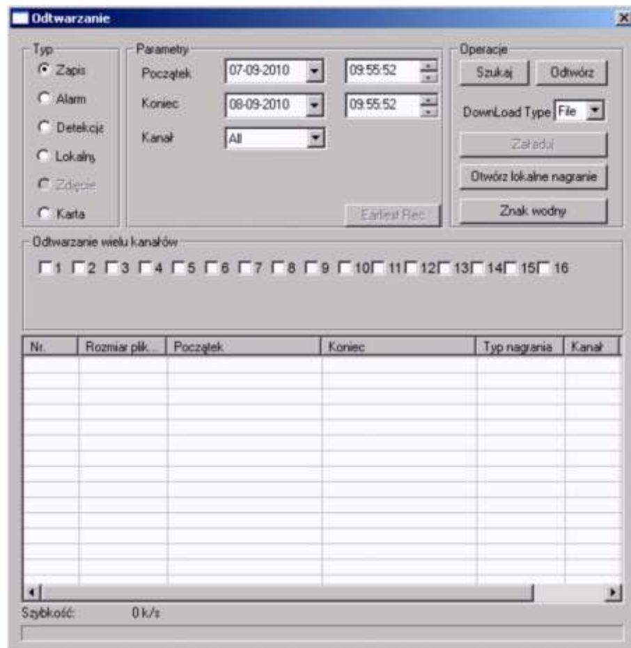
Rys. 7-58. Interfejs Wyszukiwanie.
