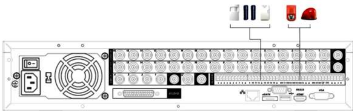
Rys. 3-5 Sposób podłączenia wejść i wyjść alarmowych.
