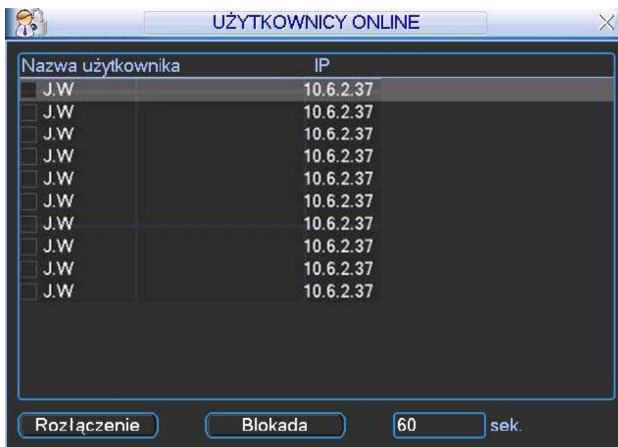
Rys. 5-46. Użytkownicy online.
