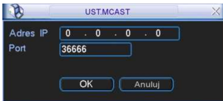
Rys. 5-11. Ustawianie MCAST.
